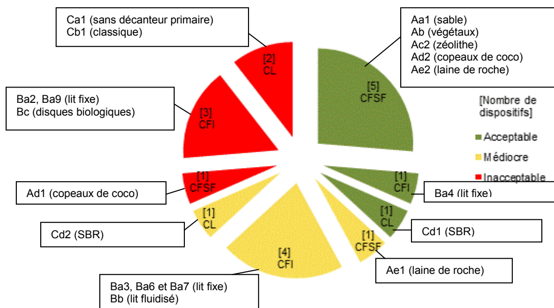
Figure 4 : Nombre de dispositifs par famille et par classe de fréquence d'entretien
