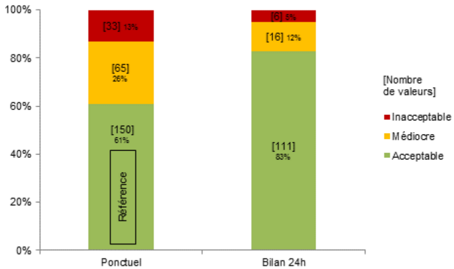
Figure 42 : Répartition dans chaque classe de qualité, selon le type de prélèvement, du paramètre MES pour la filière CFI
