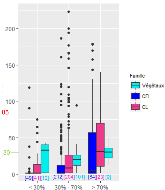
Figure 80 : Distribution des concentrations (en mg/L) du paramètre N-NH_4^+ selon les familles et le taux de charge
