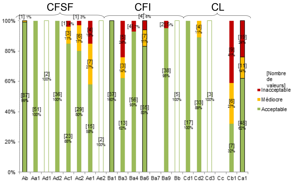
Figure 115 : Répartition dans chaque classe de qualité, selon les dispositifs, du paramètre chimique DBO 5
