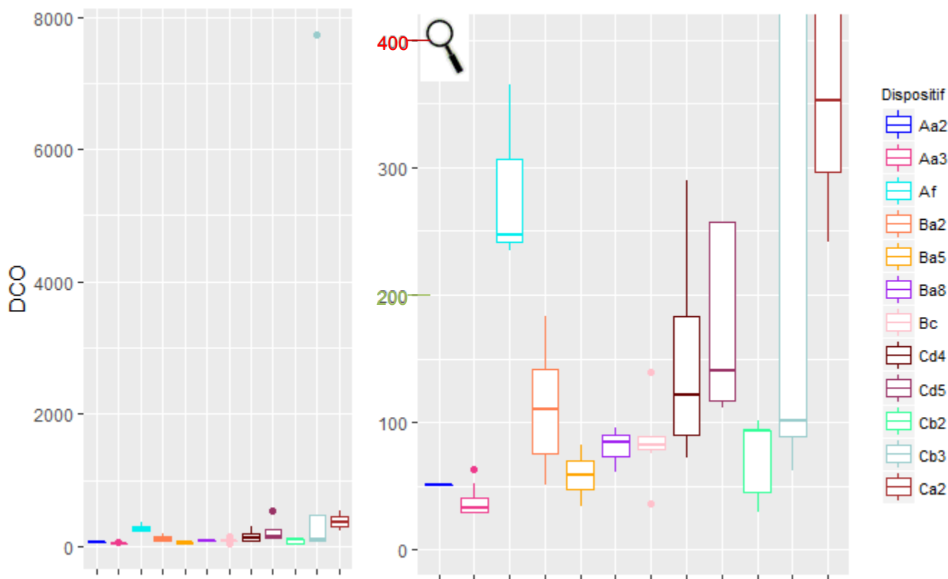
Figure 47 : Distribution des concentrations (en mg/L) du paramètre DCO selon les dispositifs (à gauche) et zoom de 0 à 400 mg/L (à droite)
