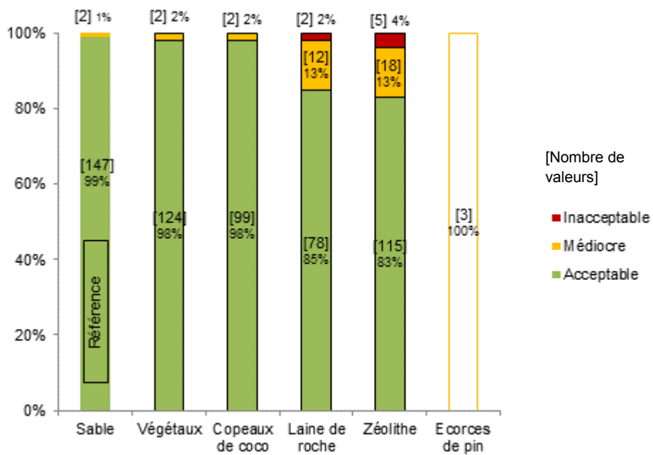
Figure 34 : Répartition dans chaque classe de qualité, selon les filières de la famille CFSF, du paramètre DCO
