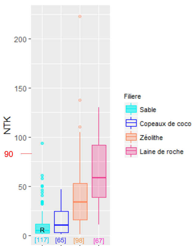
Figure 61 : Distribution des concentrations (en mg/L) du paramètre NK pour les dispositifs nitrifiants
