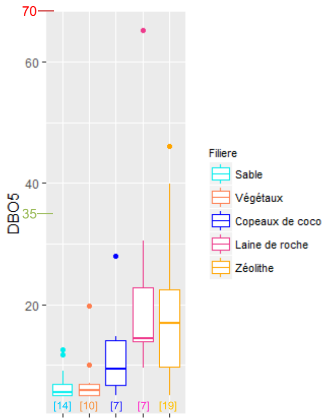
Figure 19 : Distribution des concentrations (en mg/L) du paramètre DBO 5 selon les filières de la famille CFSF
