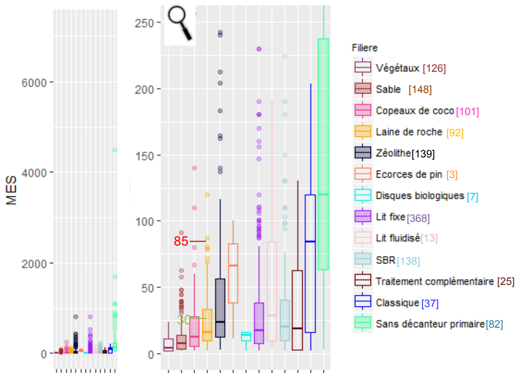
Figure 100 : Distribution des concentrations (en mg/L) du paramètre MES selon les filières (à gauche) et zoom de 0 à 250 mg/L (à droite)
