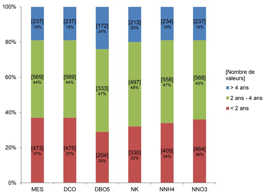
Figure 2 : Proportion de chaque paramètre chimique par classes d'âge
