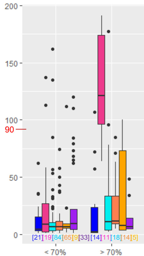
Figure 85 : Distribution des concentrations (en mg/L) du paramètre NK selon les dispositifs de la filière « lit fixe » et le taux de charge
