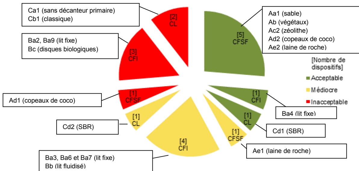
Figure 126 : Nombre de dispositifs dont les notes de l'entretien « curatif » sont « acceptable », « médiocre » ou « inacceptable » selon les familles
