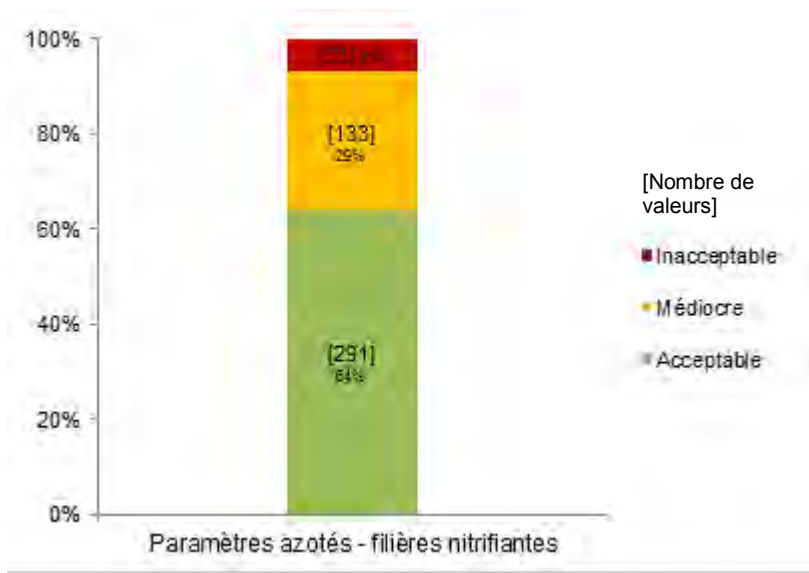
Figure 60 : Répartition, dans chaque classe de qualité, des paramètres azotés des filières nitrifiantes
