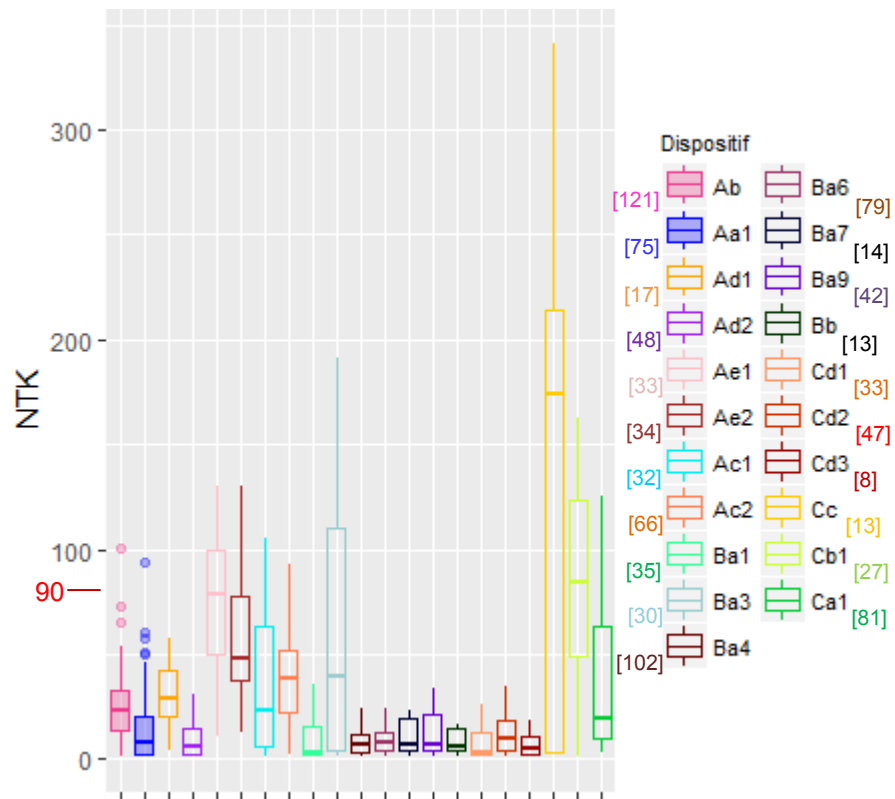
Figure 116 : Distribution des concentrations (en mg/L) du paramètre NK selon les dispositifs
