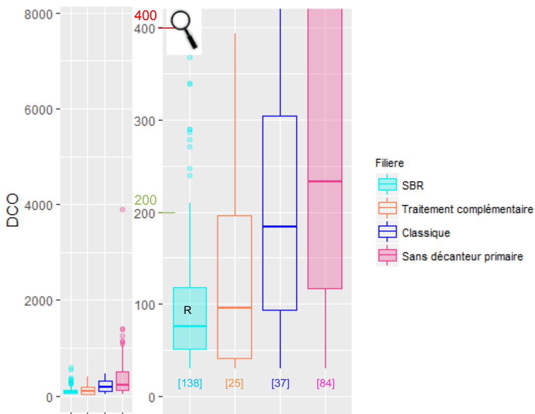
Figure 53 : Distribution des concentrations (en mg/L) du paramètre DCO selon les filières de la famille CL (à gauche) et zoom de 0 à 400 mg/L (à droite)
