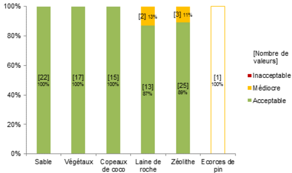
Figure 21 : Répartition dans chaque classe de qualité, selon les filières de la famille CFSF, du paramètre DCO
