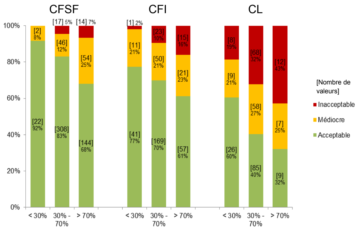
Figure 24 : Répartition dans chaque classe de qualité, selon taux de charge et familles, du paramètre MES
