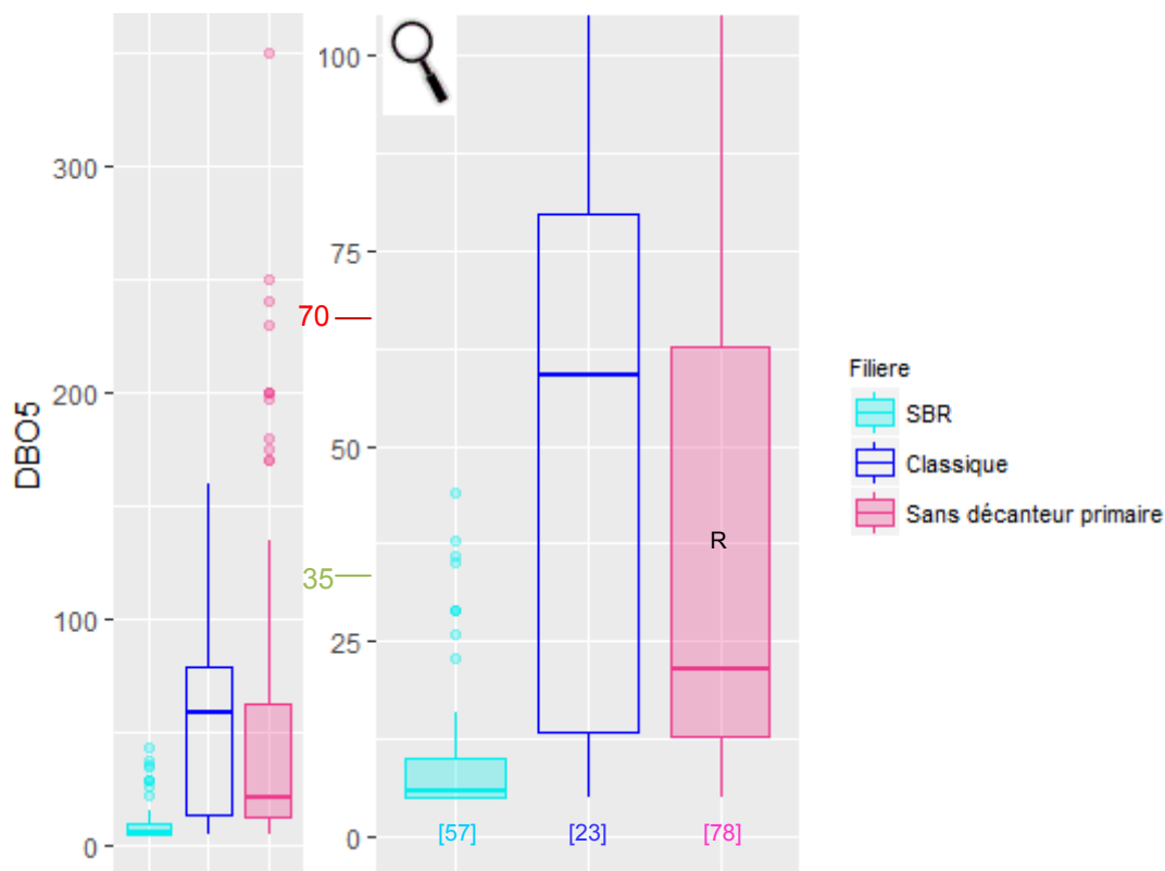
Figure 55 : Distribution des concentrations(en mg/L) du paramètre DBO_5 selon les filières de la famille CL (à gauche) et zoom de 0 à 100 mg/L (à droite)
