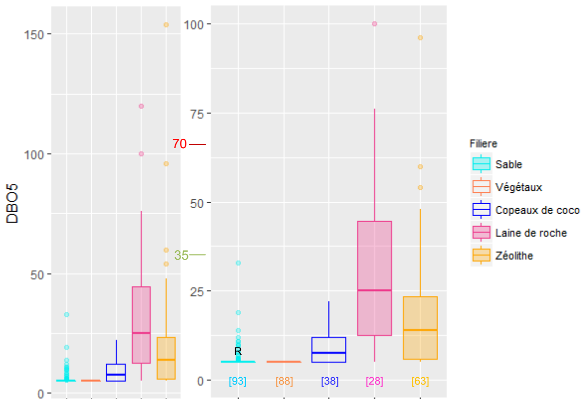
Figure 35 : Distribution des concentrations (en mg/L) du paramètre DBO 5 selon les filières de la famille CFSF (à gauche) et zoom de 0 à 100 mg/L (à droite)
