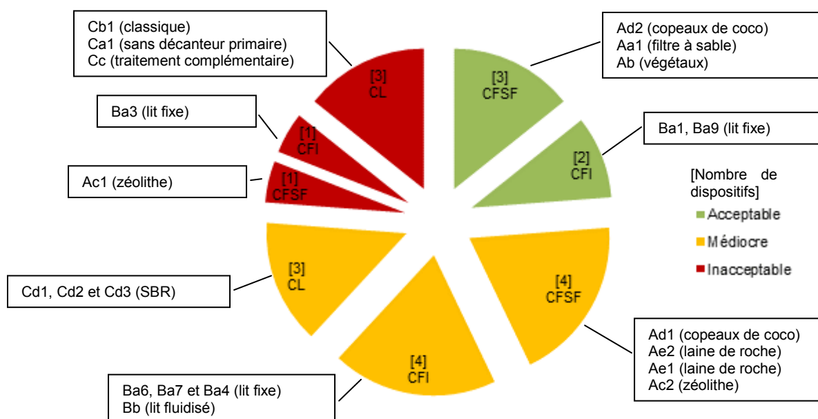
Figure 3 : Nombre de dispositifs par famille et par classe de qualité globale
