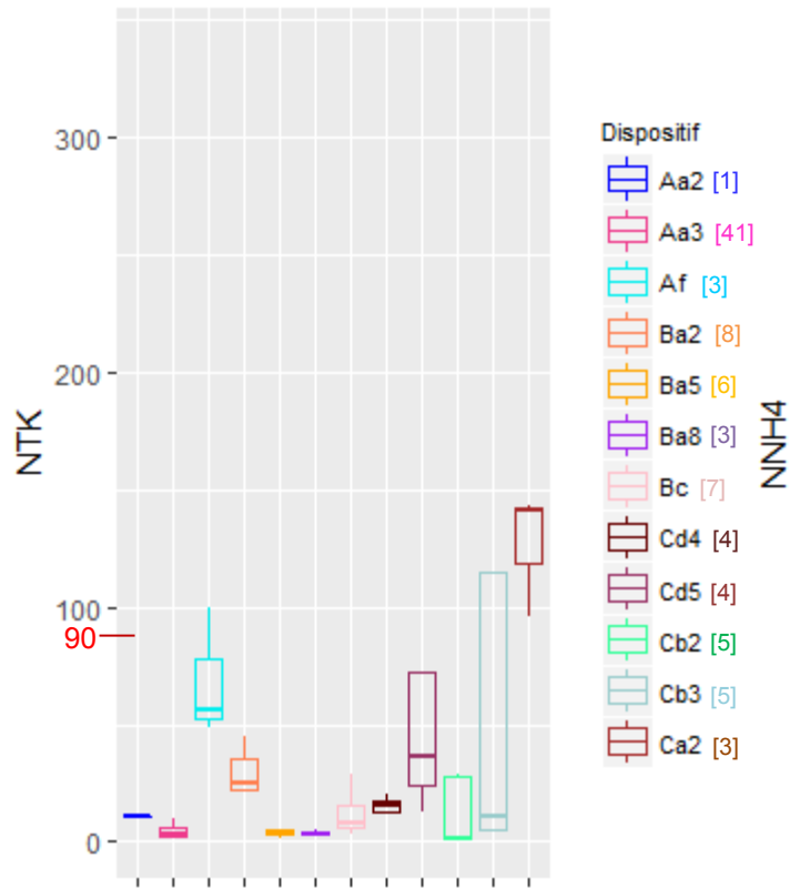
Figure 51 : Distribution des concentrations (en mg/L) du paramètre NK selon les dispositifs
