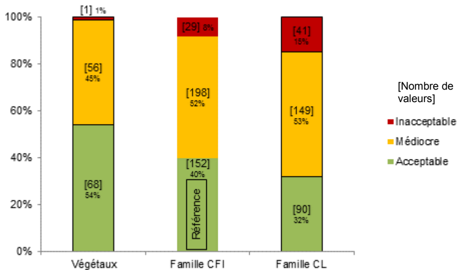
Figure 83 : Répartition dans chaque classe de qualité, selon les familles nitrifiants-dénitrifiants, des paramètres caractéristiques de l'azote
