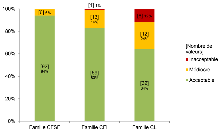
Figure 11 : Répartition dans chaque classe de qualité, selon les familles, du paramètre DCO
