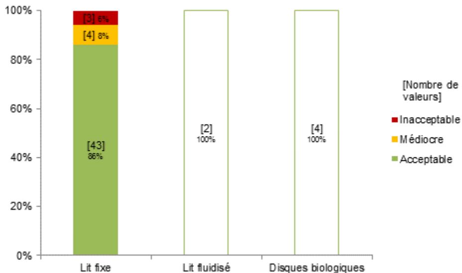
Figure 31 : Répartition dans chaque classe de qualité, selon les filières de la famille CFI, du paramètre DBO 5
