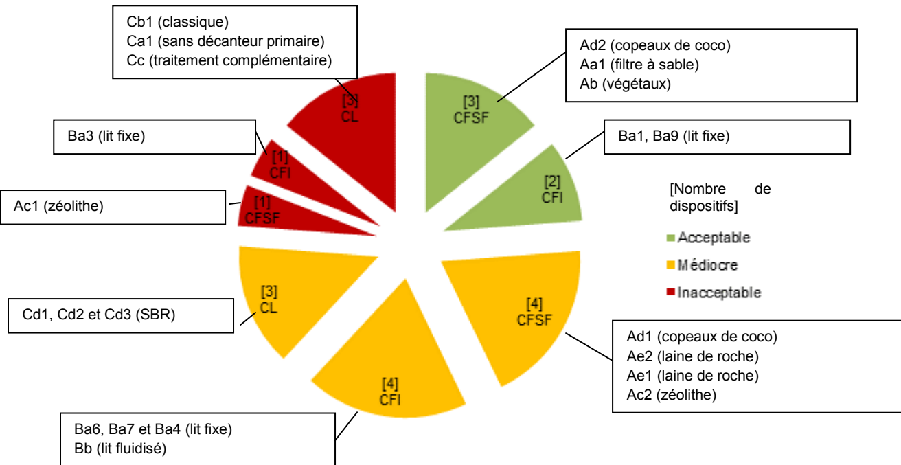
Figure 120 : Nombre de dispositifs par famille et par classe de qualité
