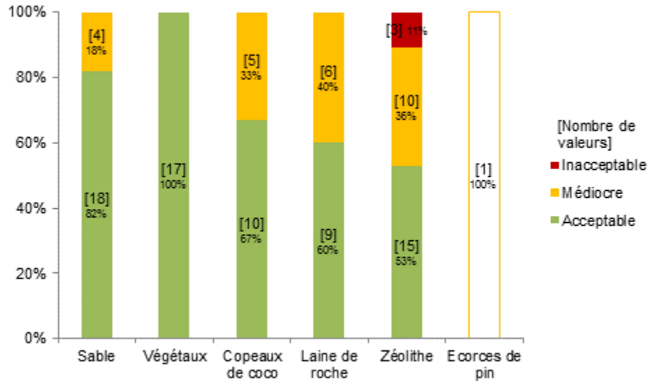
Figure 20 : Répartition dans chaque classe de qualité, selon les filières de la famille CFSF, du paramètre MES
