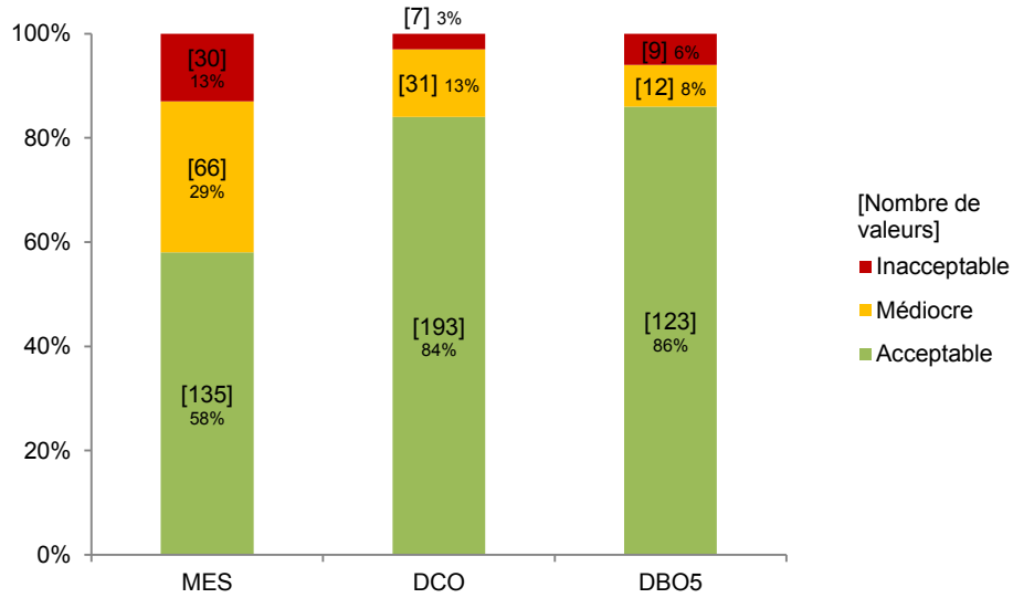
Figure 7 : Répartition, dans chaque classe de qualité, des trois paramètres MES, DCO et DBO 5 (ensemble des données)
