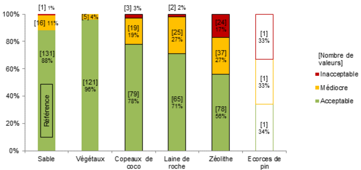
Figure 32 : Répartition dans chaque classe de qualité, selon les filières de la famille CFSF, du paramètre MES
