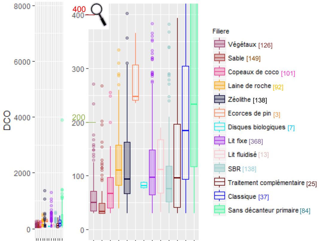
Figure 102 : Distribution des concentrations (en mg/L) du paramètre DCO selon les filières (à gauche) et zoom de 0 à 400 mg/L (à droite)
