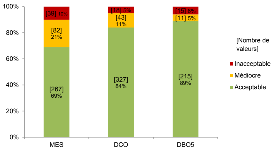
Figure 41 : Répartition, dans chaque classe de qualité, des trois paramètres MES, DCO et DBO 5 (famille CFI)
