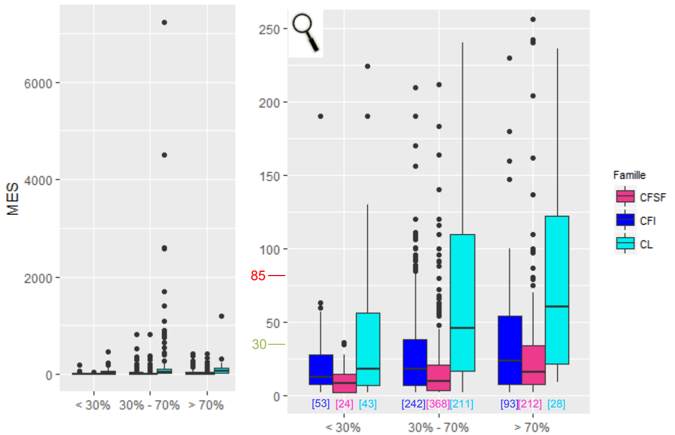
Figure 23 : Distribution des concentrations (en mg/L) du paramètre MES selon le taux de charge et par famille (à gauche) et zoom de 0 à 250 mg/L (à droite)
