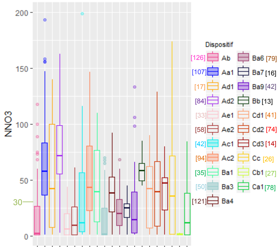
Figure 118 : Distribution des concentrations (en mg/L) du paramètre N-NO3- selon les dispositifs
