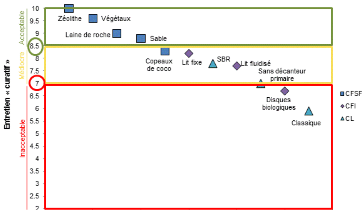
Figure 128 : Notes d'entretien « curatif » de 11 filières par ordre décroissant
