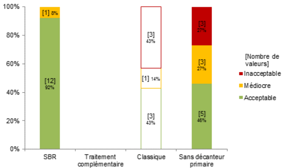
Figure 40 : Répartition dans chaque classe de qualité, selon les filières de la famille CL, du paramètre DBO 5
