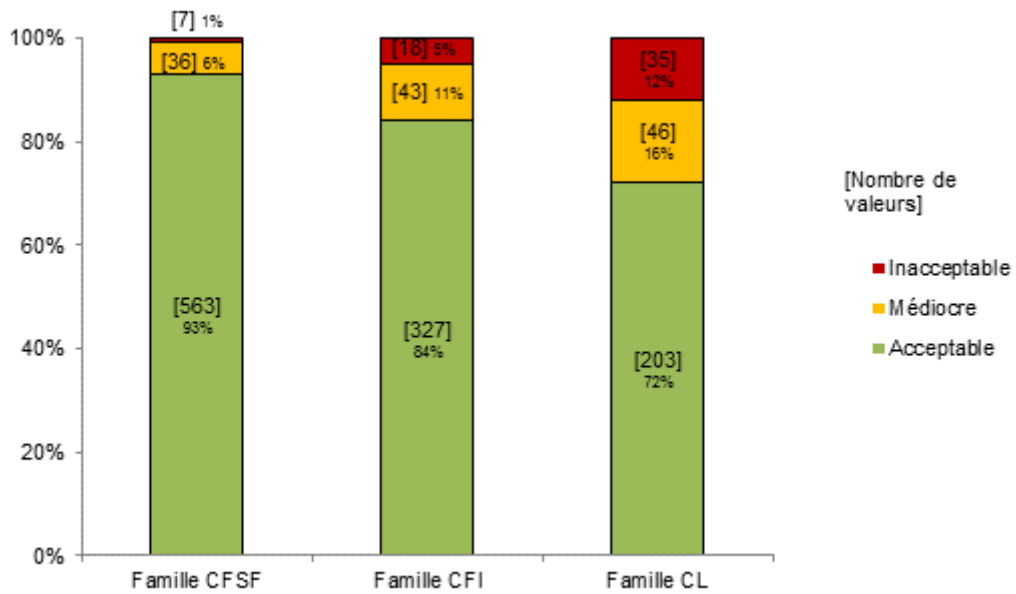
Figure 93 : Répartition dans chaque classe de qualité, selon les familles, du paramètre chimique DCO
