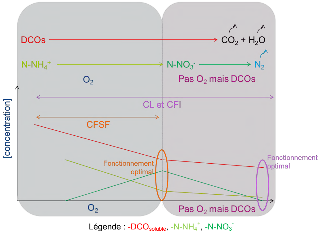
Figure 4 : Représentation schématique du traitement de la pollution dissoute
