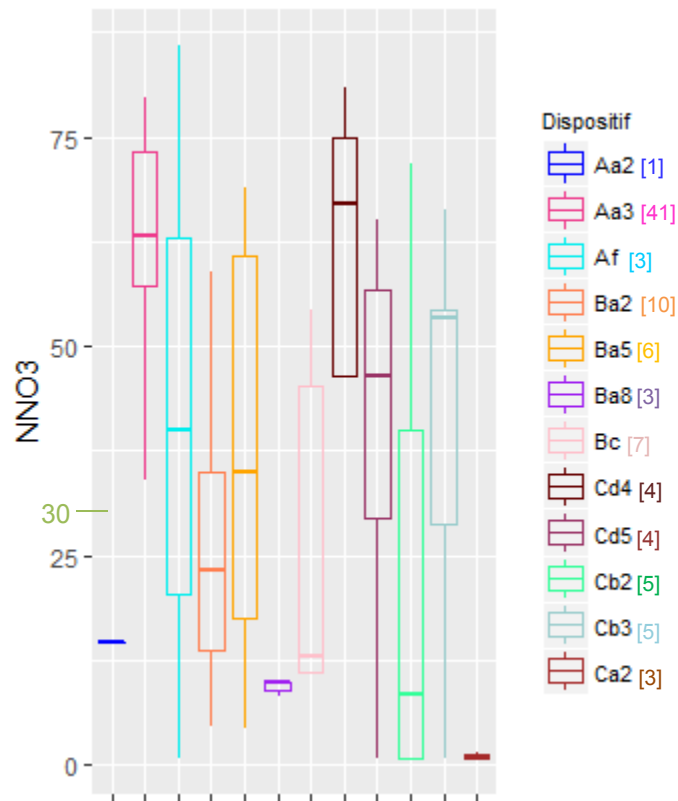
Figure 53 : Distribution des concentrations (en mg/L) du paramètre N-NO_3^- selon les dispositifs
