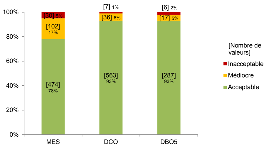
Figure 30 : Répartition, dans chaque classe de qualité, des trois paramètres MES, DCO et DBO 5 (famille CFSF)
