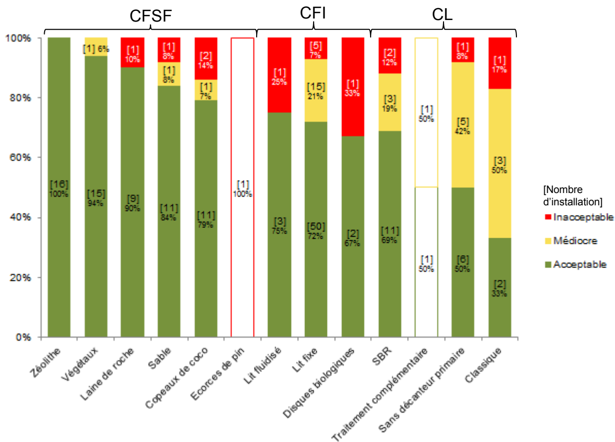
Figure 122 : Répartition des installations par filière selon leurs fréquences « acceptable », « médiocre » ou « inacceptable » de l'entretien « curatif »
