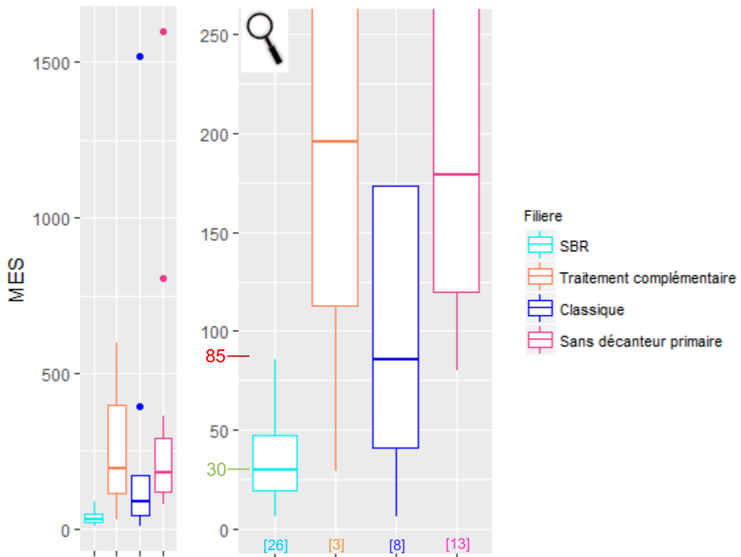
Figure 35: Distribution des concentrations (en mg/L) du paramètre MES selon les filières de la famille CL (à gauche) et zoom de 0 à 250 mg/L (à droite)
