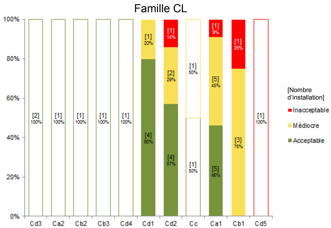
Figure 125 : Répartition des installations des CL par dispositif selon leurs fréquences « acceptable », « médiocre » ou « inacceptable » de l'entretien « curatif »
