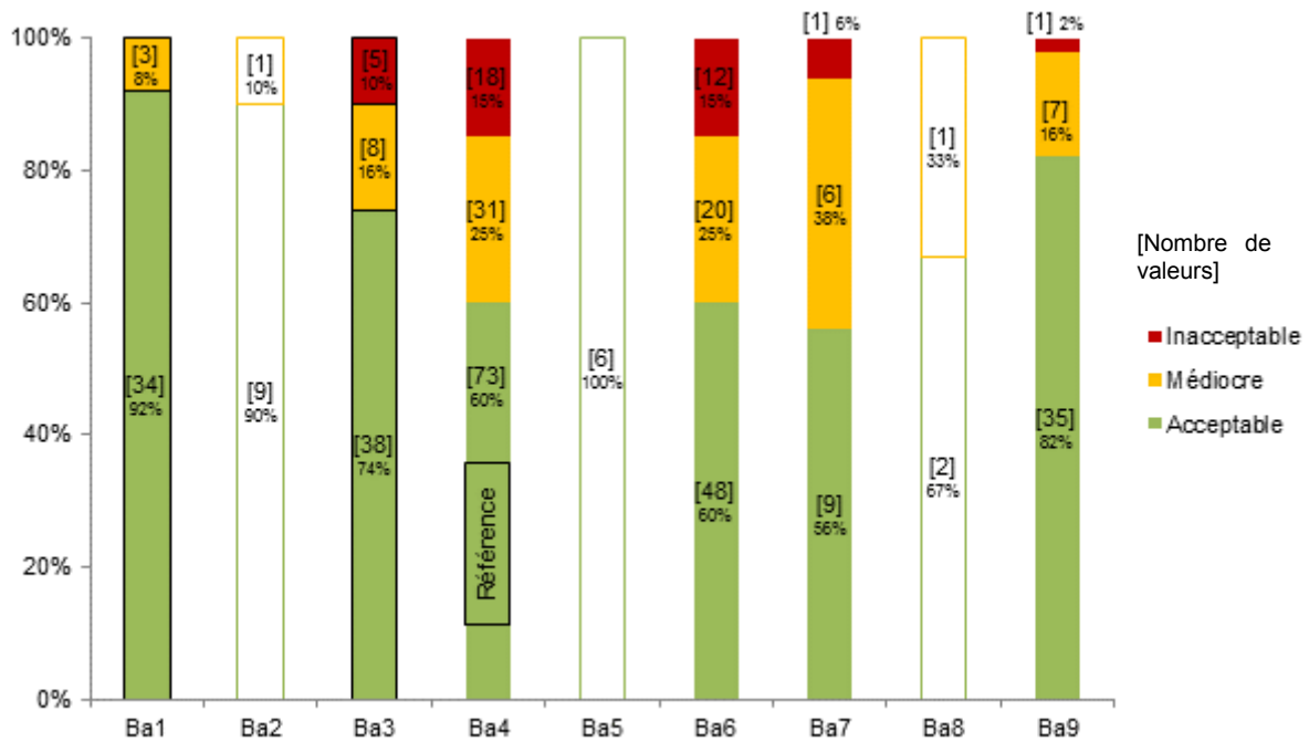
Figure 43 : Répartition dans chaque classe de qualité, selon les dispositifs de la filière « lit fixe », du paramètre MES
