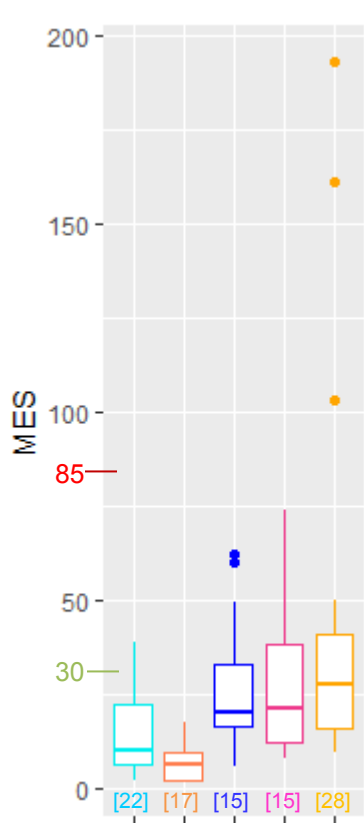
Figure 17 : Distribution des concentrations (en mg/L) du paramètre MES selon les filières de la famille CFSF
