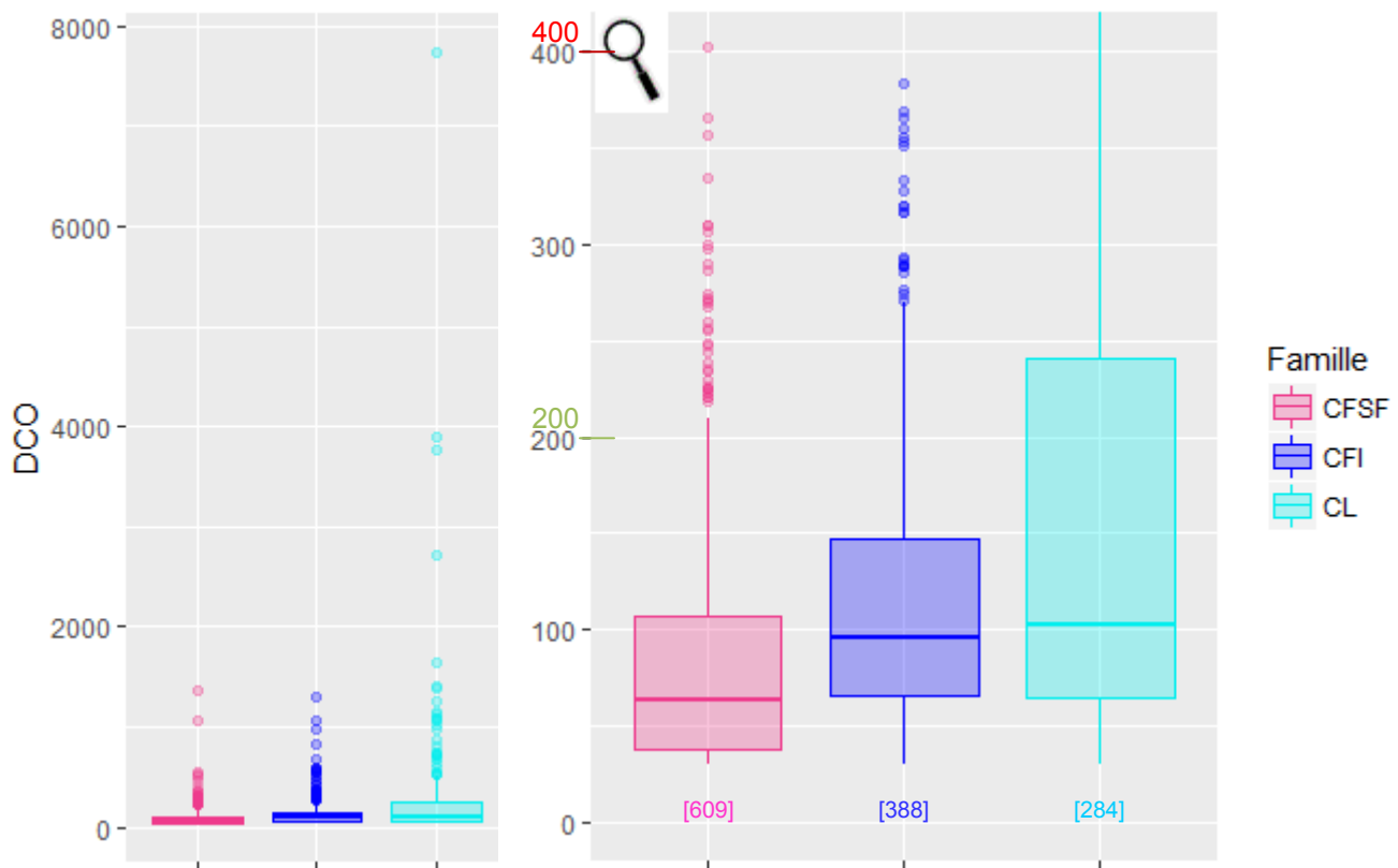
Figure 92 : Distribution des concentrations (en mg/L) du paramètre DCO selon les familles (à gauche) et zoom de 0 à 400 mg/L (à droite)
