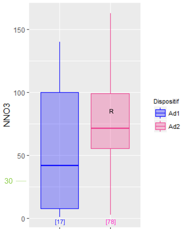
Figure 72 : Distribution des concentrations (en mg/L) du paramètre chimique N-NO_3^- selon les dispositifs de la filière « copeaux de coco »
