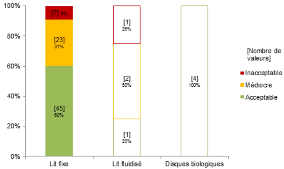
Figure 29 : Répartition dans chaque classe de qualité, selon les filières de la famille CFI, du paramètre MES
