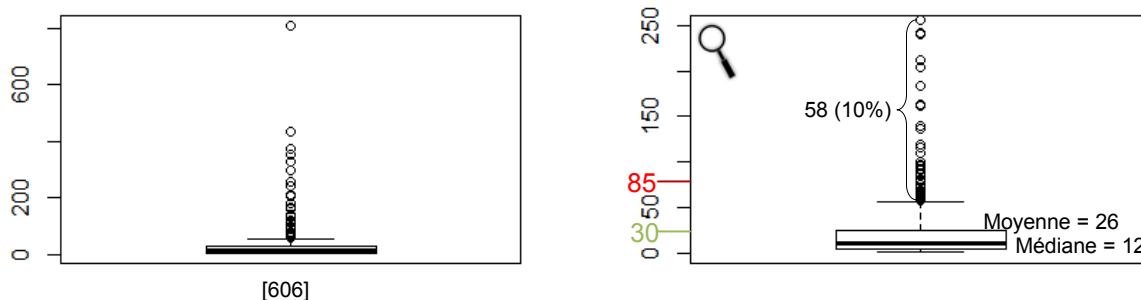
Figure 28 : Distribution des concentrations (en mg/L) du paramètre MES pour la famille CFSF (à gauche) et zoom de 0 à 250 mg/L (à droite)
