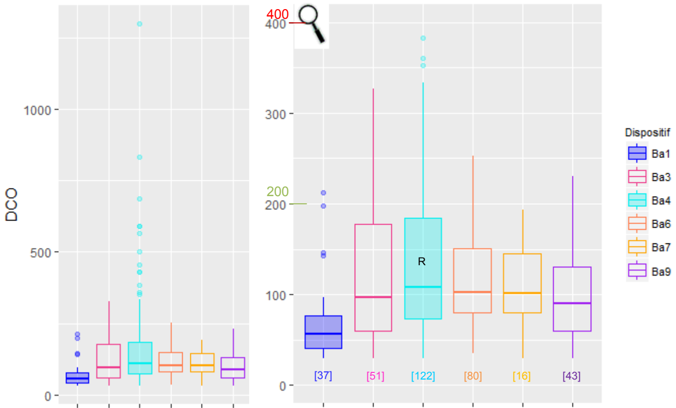
Figure 44 : Distribution des concentrations (en mg/L) du paramètre DCO selon les dispositifs de la famille CFI (à gauche) et zoom de 0 à 400 mg/L (à droite)
