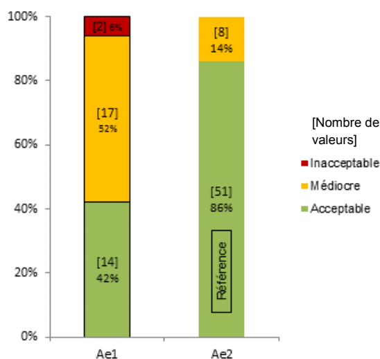
Figure 38 : Répartition, dans chaque classe de qualité, du paramètre MES (deux dispositifs de la filière « laine de roche »)
