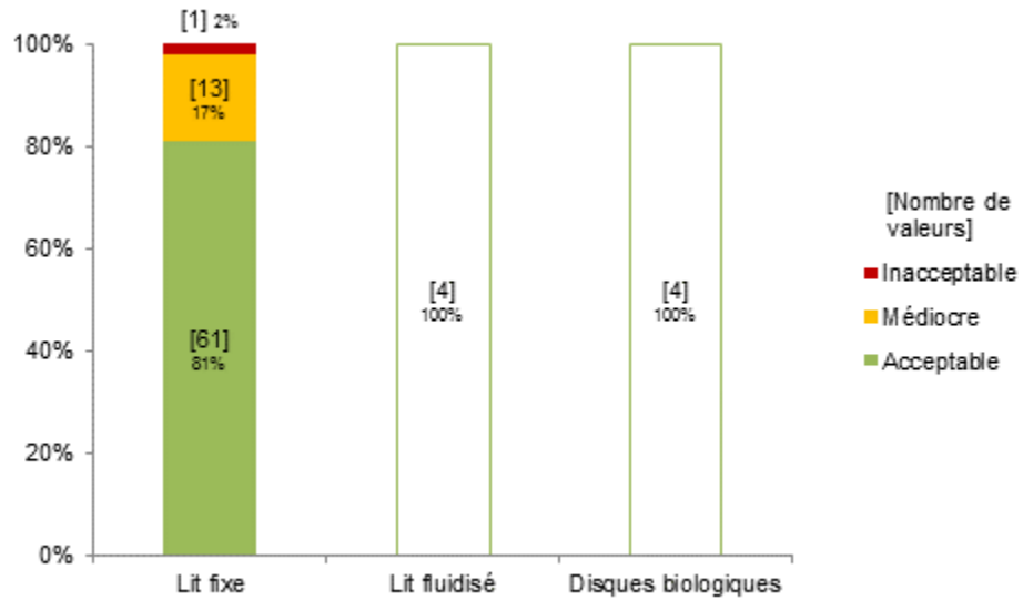
Figure 29 : Répartition dans chaque classe de qualité, selon les filières de la famille CFI, du paramètre MES
