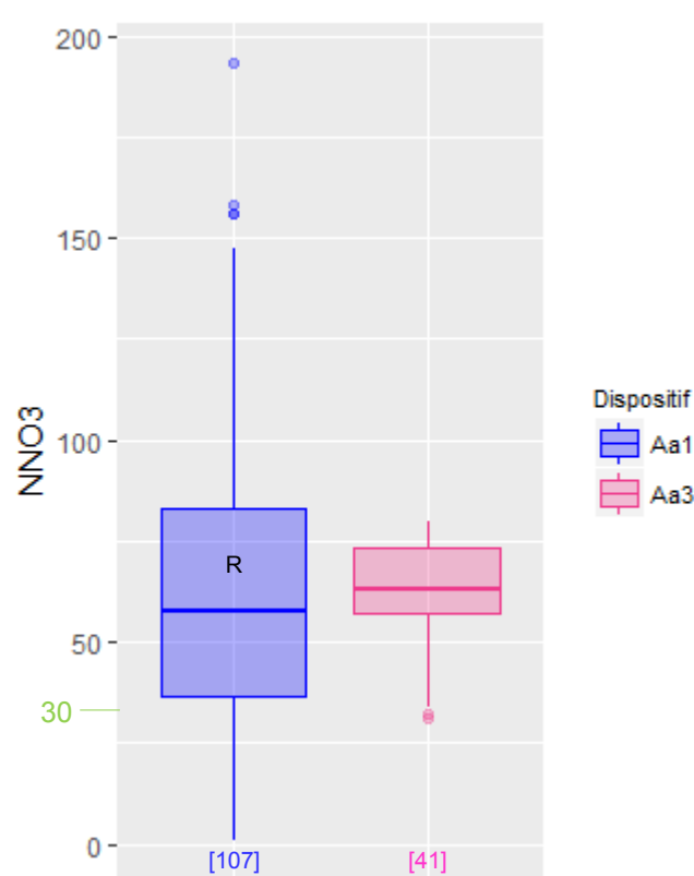
Figure 68 : Distribution des concentrations (en mg/L) du paramètre N-NO 3 - selon les dispositifs de la filière « sable »
