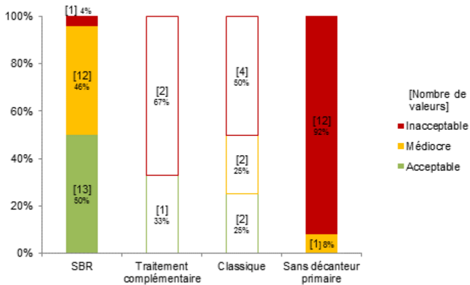
Figure 36 : Répartition dans chaque classe de qualité, selon les filières de la famille CL, du paramètre MES
