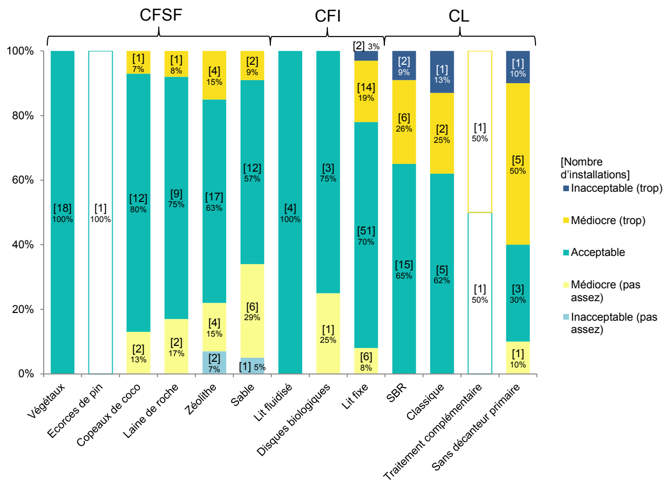
Figure 56 : Répartition des installations par filière selon leurs fréquences de vidange « acceptable », « médiocre » (trop ou pas assez) ou « inacceptable » (trop ou pas assez)
