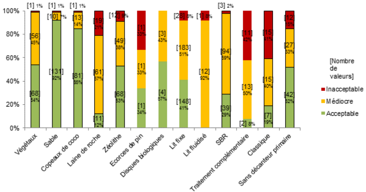
Figure 109 : Répartition dans chaque classe de qualité, selon les filières, des paramètres azotés
