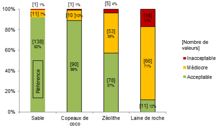
Figure 63 : Distribution des concentrations (en mg/L) du paramètre N-NO_3^- pour les dispositifs nitrifiants
