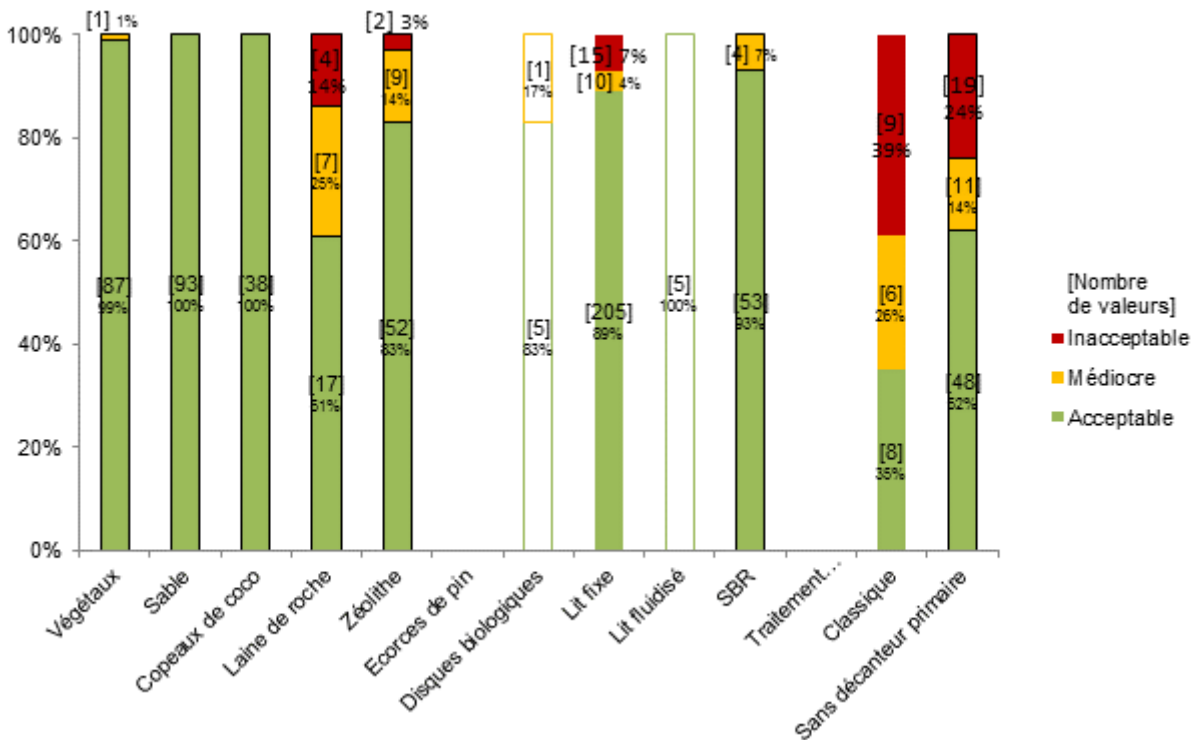
Figure 105 42 : Répartition dans chaque classe de qualité, selon les filières, du paramètre chimique DBO 5
