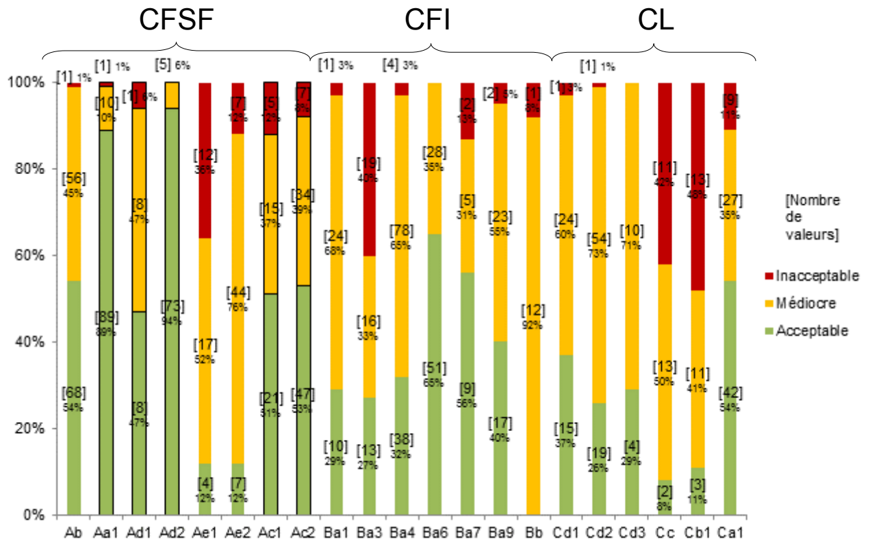
Figure 119 : Répartition dans chaque classe de qualité, selon les dispositifs, des paramètres azotés
