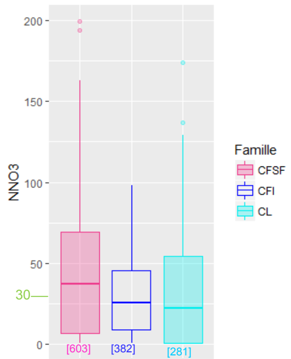
Figure 98 : Distribution des concentrations (en mg/L) du paramètre N-NO 3 - selon les familles
