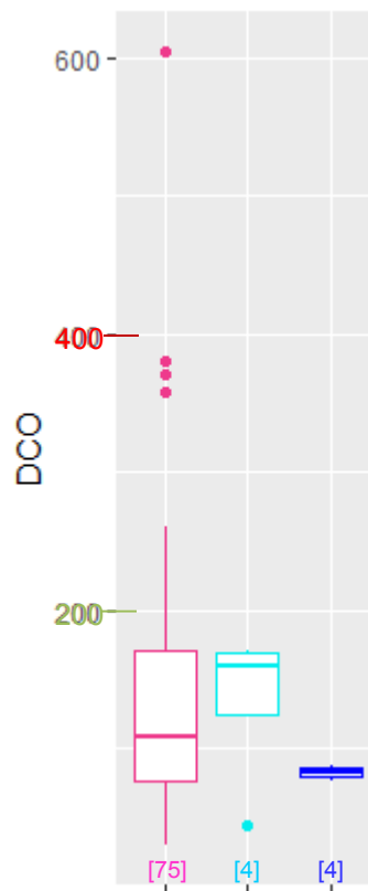
Figure 27 : Distribution des concentrations (en mg/L) du paramètre DCO selon les filières de la famille CFI
