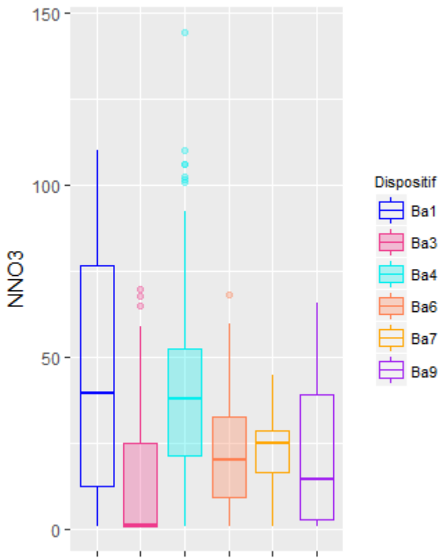
Figure 87 : Distribution des concentrations (en mg/L) du paramètre N-NO_3^- selon les dispositifs de la filière « lit fixe »
