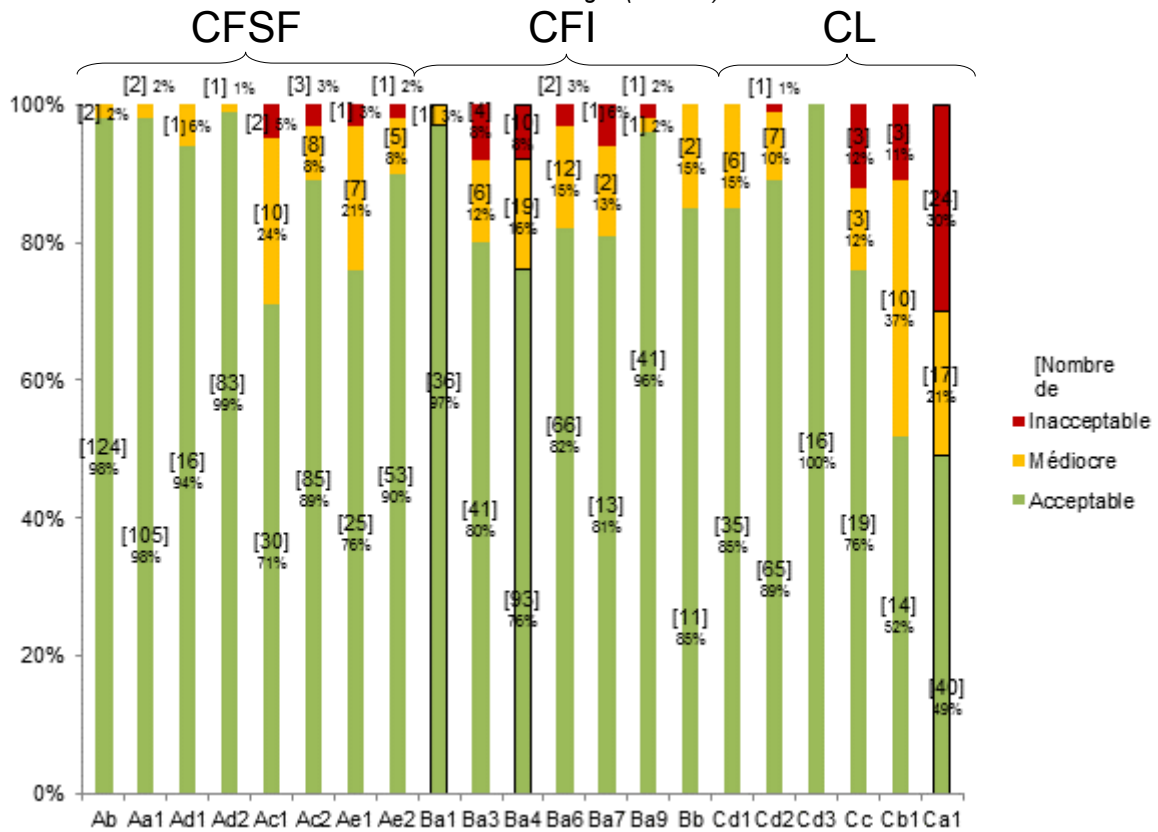
Figure 113 : Répartition dans chaque classe de qualité, selon les dispositifs, du paramètre chimique DCO
