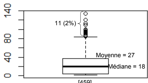
Figure 58 : Distribution des concentrations (en mg/L) du paramètre N-NH 4 + des filières nitrifiantes
