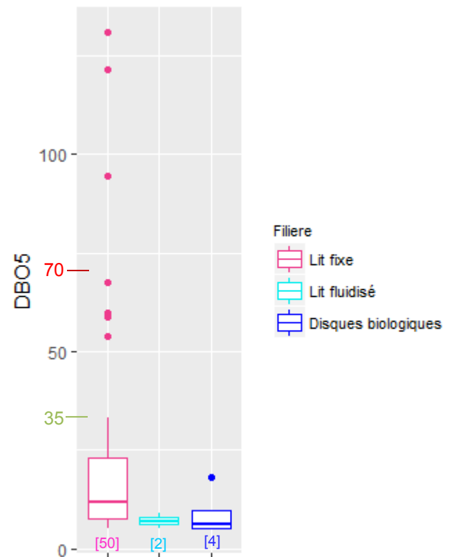
Figure 28 : Distribution des concentrations (en mg/L) du paramètre DBO 5 selon les filières de la famille CFI
