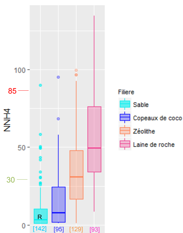
Figure 62 : Distribution des concentrations (en mg/L) du paramètre N-NH_4^+ pour les dispositifs nitrifiants
