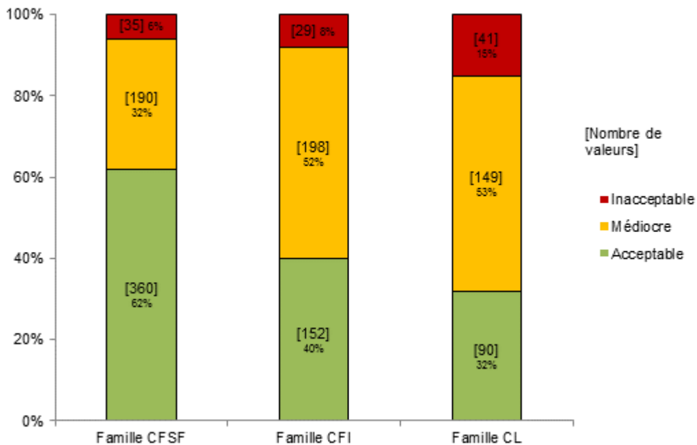
Figure 99 : Répartition dans chaque classe de qualité, selon les familles, des paramètres azotés
