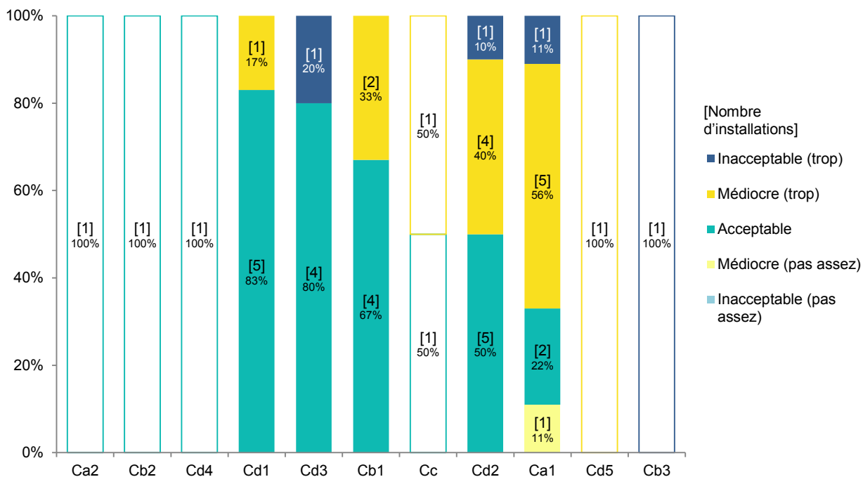
Figure 59 : Répartition des installations des CL par dispositif selon leurs fréquences de vidange « acceptable », « médiocre » (trop ou pas assez) ou « inacceptable » (trop ou pas assez)
