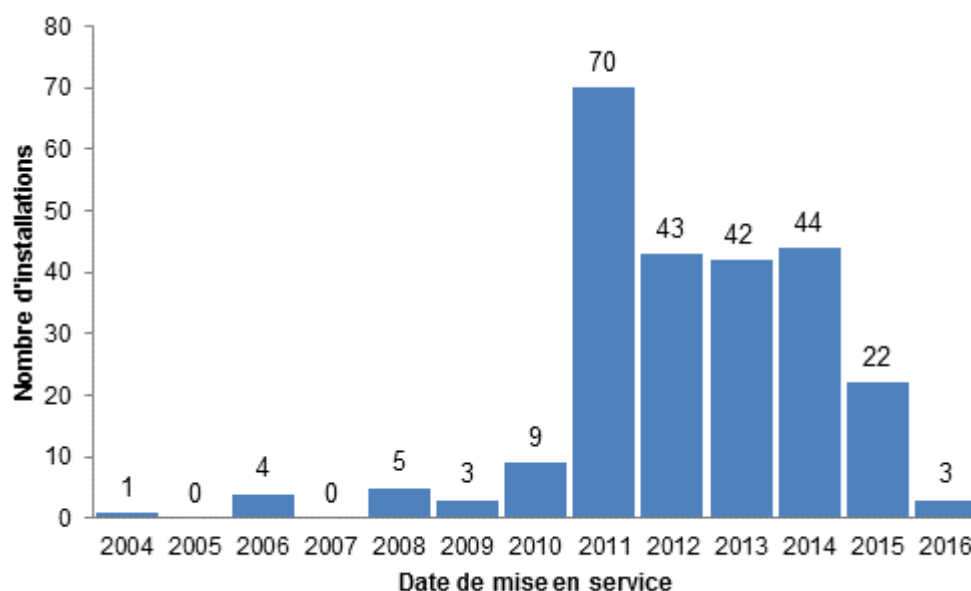
Figure 11 : Date de mise en service des installations suivies
