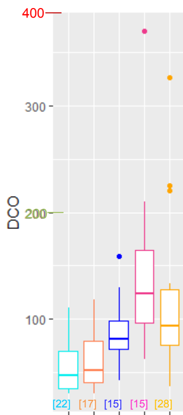
Figure 18 : Distribution des concentrations (en mg/L) du paramètre DCO selon les filières de la famille CFSF
