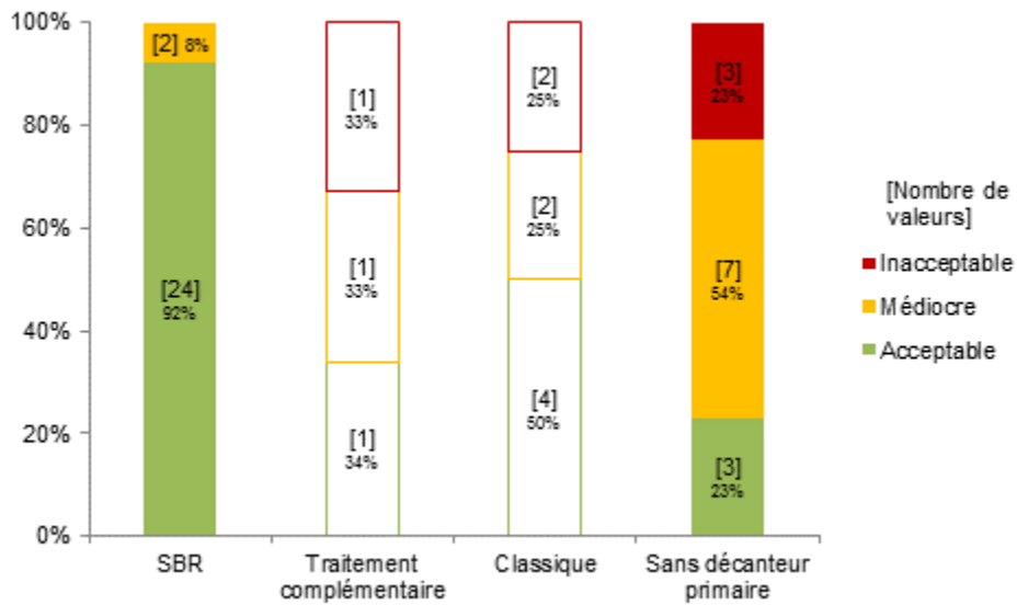
Figure 38 : Répartition dans chaque classe de qualité, selon les filières de la famille CL, du paramètre DCO
