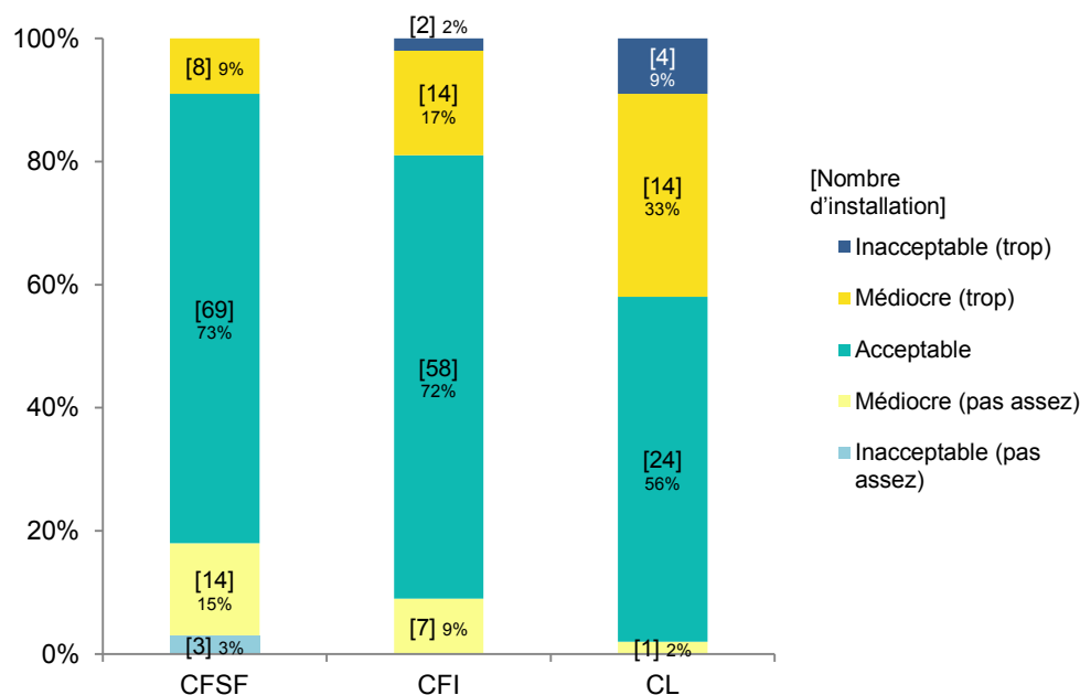
Figure 55 : Répartition des installations par famille selon leurs fréquences de vidange « acceptable », « médiocre » (trop ou pas assez) ou « inacceptable » (trop ou pas assez)
