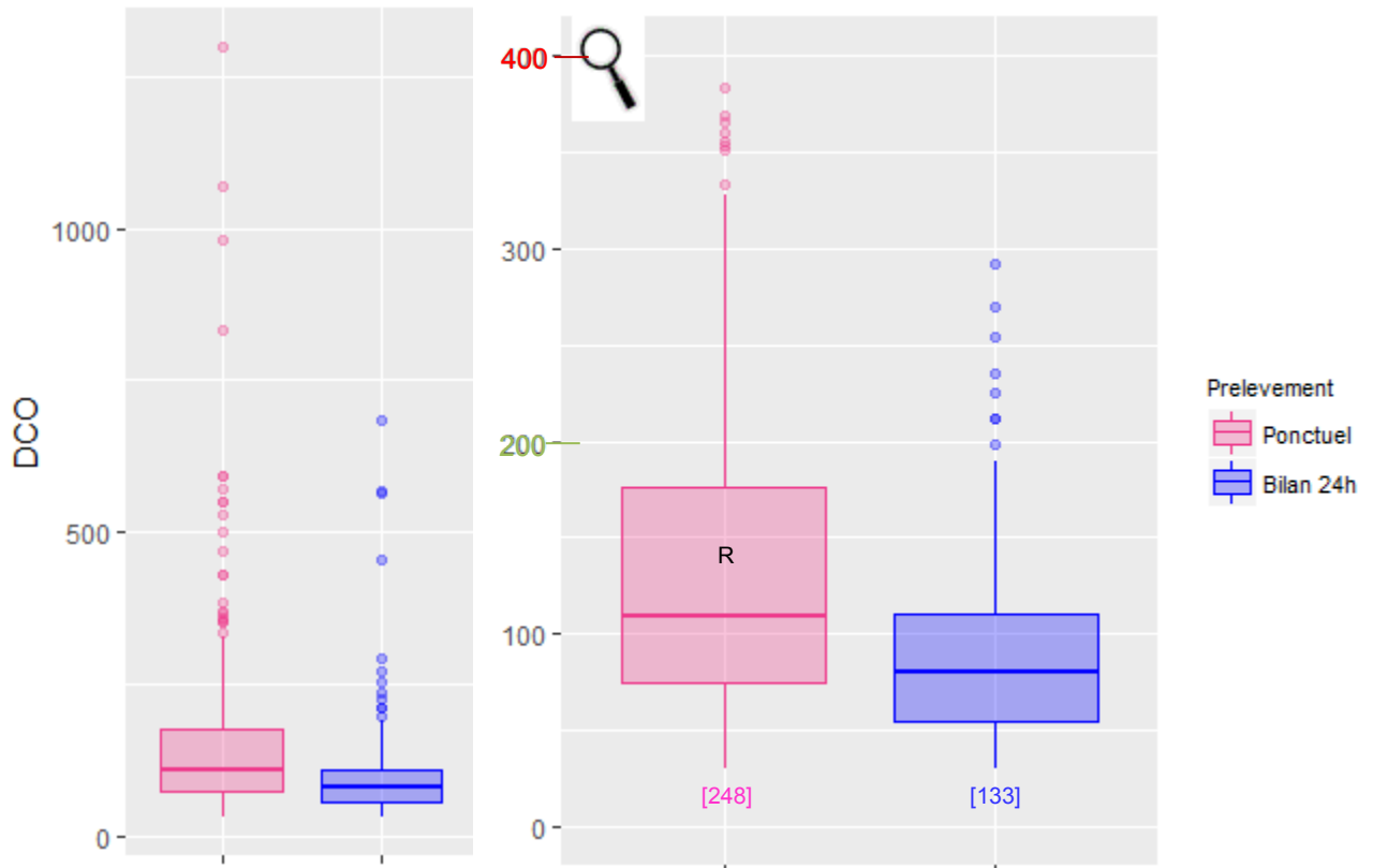
Figure 43 : Distribution des concentrations (en mg/L) du paramètre DCO selon le type de prélèvement (à gauche) et zoom de 0 à 400 mg/L (à droite) pour les filières de la famille CFI
