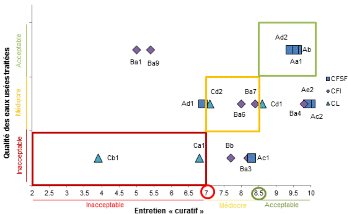
Figure 5 : Analyse conjointe de la qualité des eaux usées traitées et de l'entretien « curatif » des 18 dispositifs
