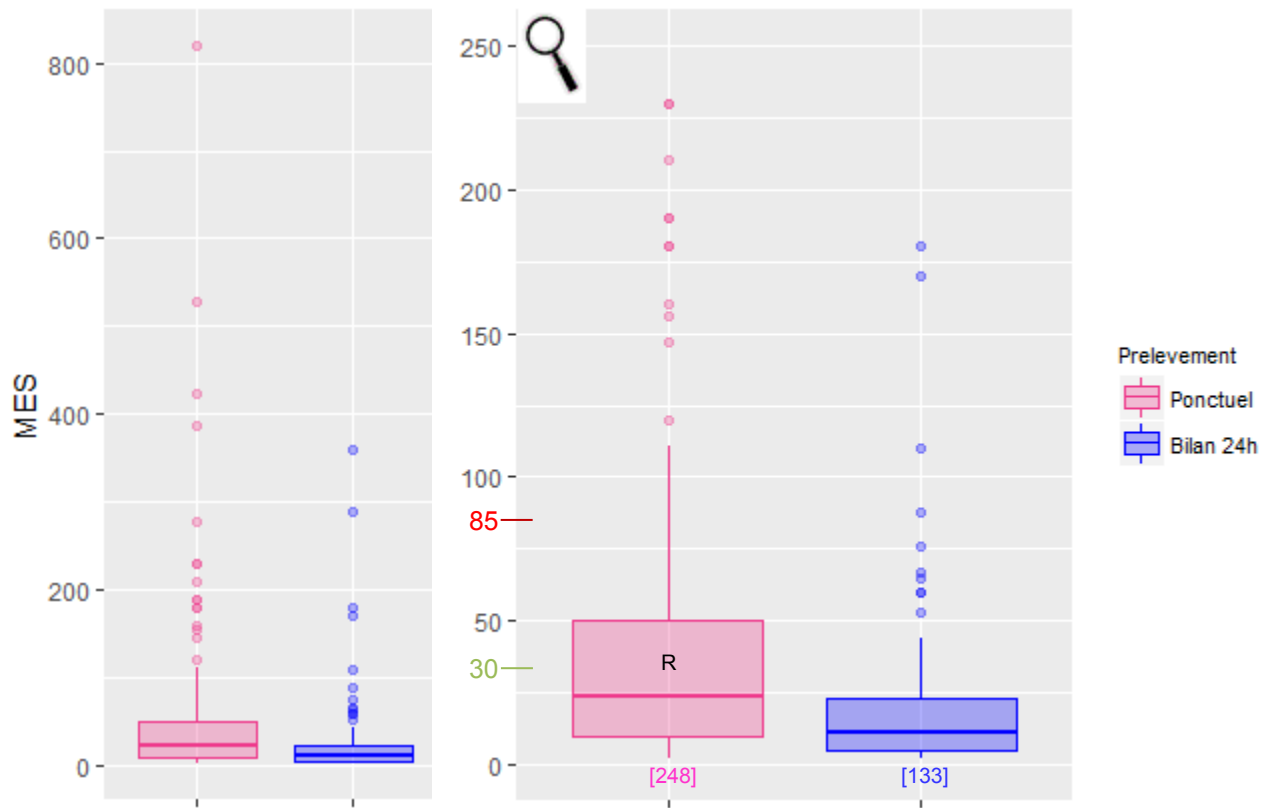
Figure 41 : Distribution des concentrations (en mg/L) du paramètre MES selon le type de prélèvement (à gauche) et zoom de 0 à 250 mg/L (à droite) pour les filières de la famille CFI
