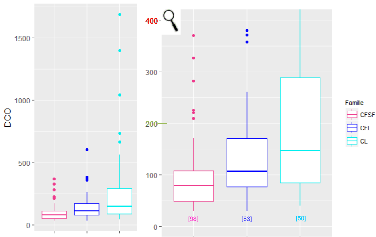
Figure 10 : Distribution des concentrations (en mg/L) du paramètre DCO selon les familles (à gauche) et zoom de 0 à 400 mg/L (à droite)
