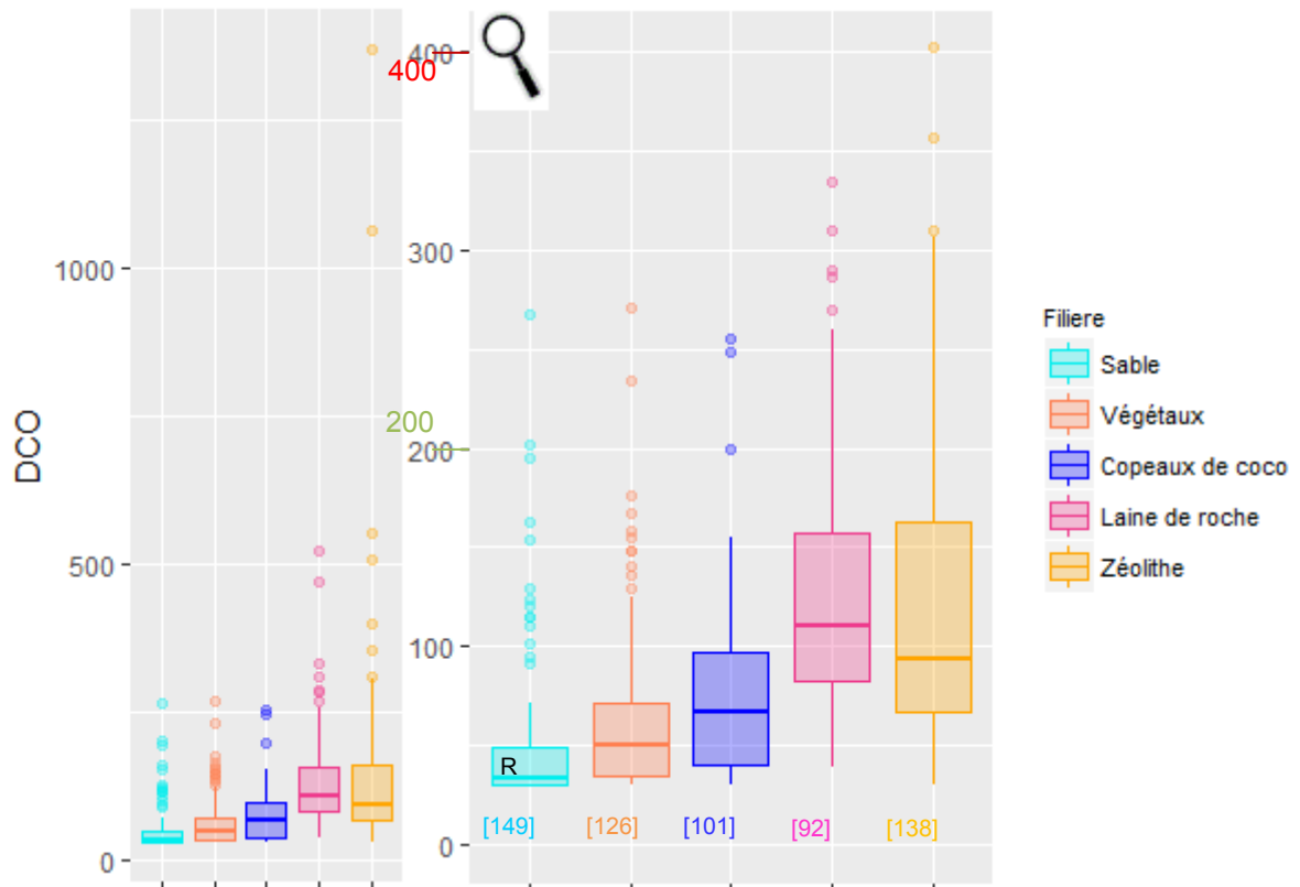
Figure 33 : Distribution des concentrations (en mg/L) du paramètre DCO selon les filières de la famille CFSF (à gauche) et zoom de 0 à 400 mg/L (à droite)
