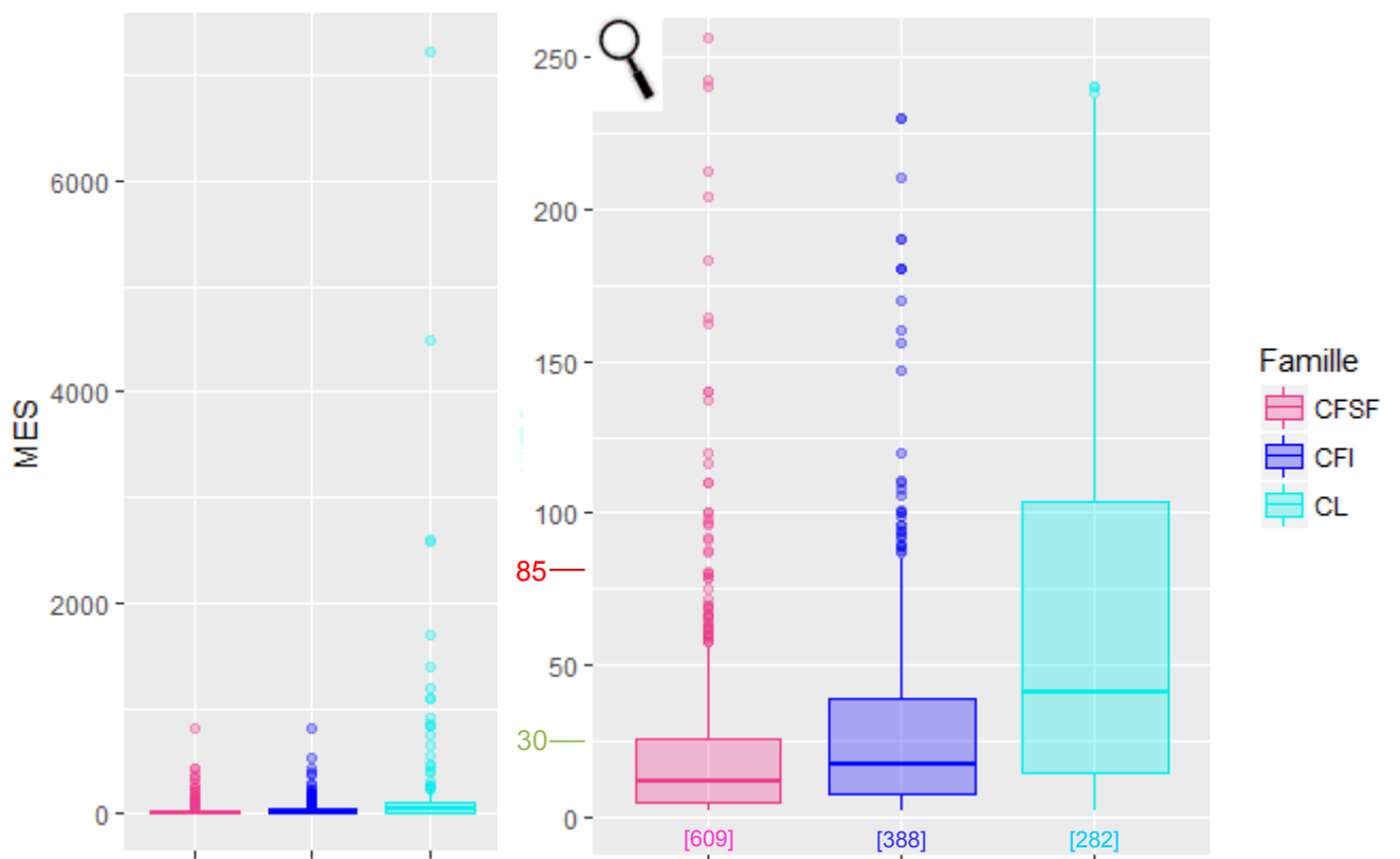
Figure 90 : Distribution des concentrations (en mg/L) du paramètre MES selon les familles (à gauche) et zoom de 0 à 250 mg/L (à droite)
