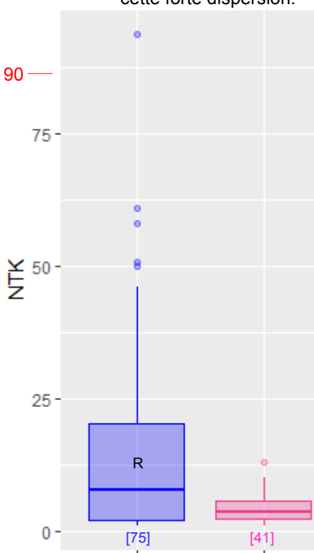
Figure 66 : Distribution des concentrations (en mg/L) du paramètre NK selon les dispositifs de la filière « sable »
