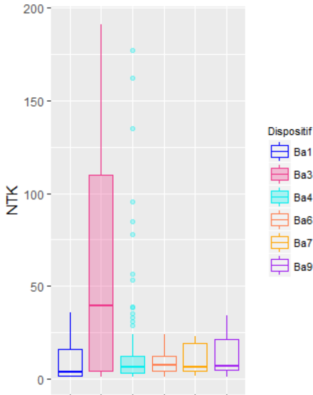
Figure 84 : Distribution des concentrations (en mg/L) du paramètre NK selon les dispositifs de la filière « lit fixe »
