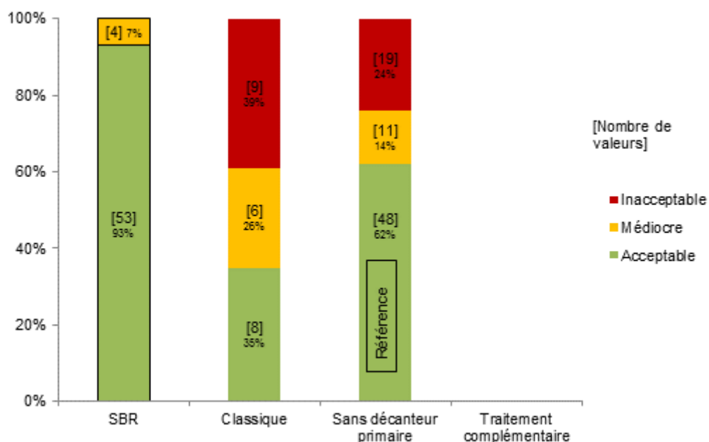
Figure 56 : Répartition dans chaque classe de qualité, selon les filières de la famille CL, du paramètre DBO_5
