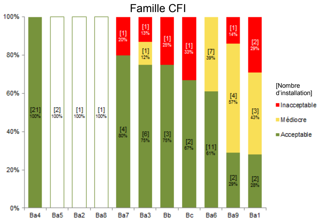
Figure 124 : Répartition des installations des CFI par dispositif selon leurs fréquences « acceptable », « médiocre » ou « inacceptable » de l'entretien « curatif »
