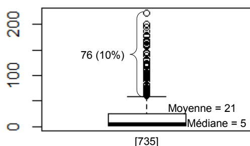
Figure 74 : Distribution de toutes les concentrations (en mg/L) du paramètre N-NH_4^+ des dispositifs nitrifiants-dénitrifiants
