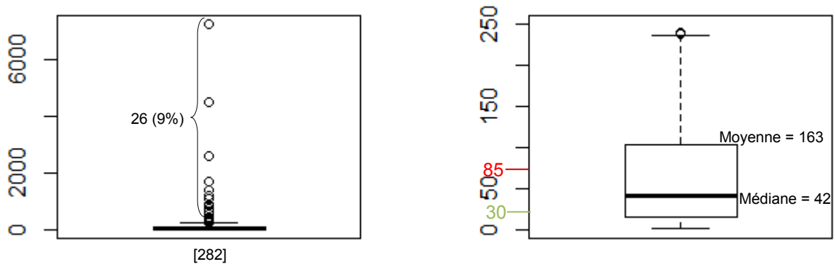
Figure 48 : Distribution des concentrations (en mg/L) du paramètre MES de la famille CL (à gauche) et zoom de 0 à 250 mg/L (à droite)
