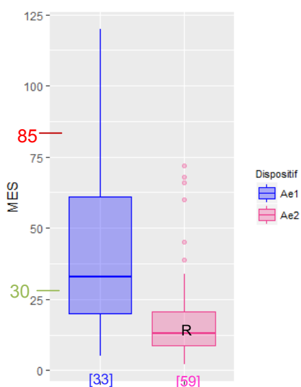
Figure 37 : Distribution des concentrations (en mg/L) du paramètre MES (deux dispositifs de la filière « laine de roche »)
