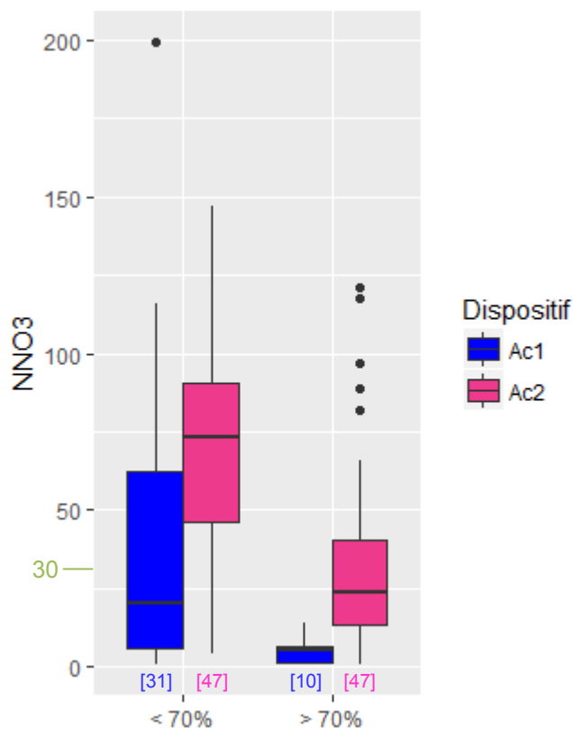
Figure 70 : Distribution des concentrations (en mg/L) du paramètre N-NO_3^- selon les deux dispositifs de la filière « zéolithe » et le taux de charge
