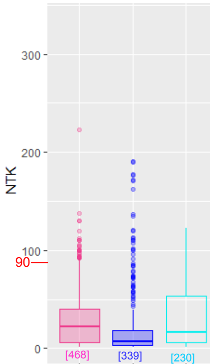
Figure 96 : Distribution des concentrations (en mg/L) du paramètre NK selon les familles
