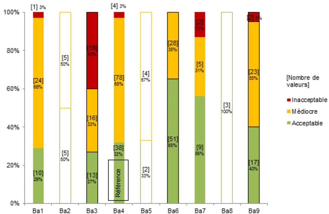
Figure 89 : Répartition dans chaque classe de qualité, selon les dispositifs de la filière « lit fixe », des paramètres caractéristiques de l'azote
