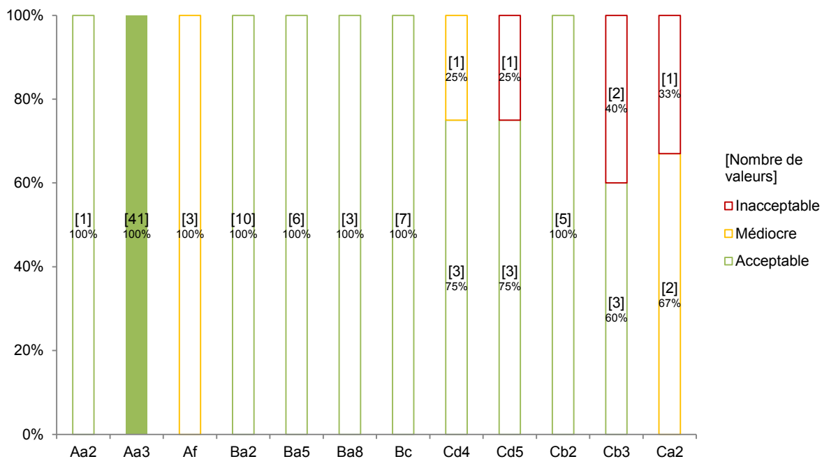
Figure 48 : Répartition dans chaque classe de qualité, selon les dispositifs, du paramètre chimique DCO
