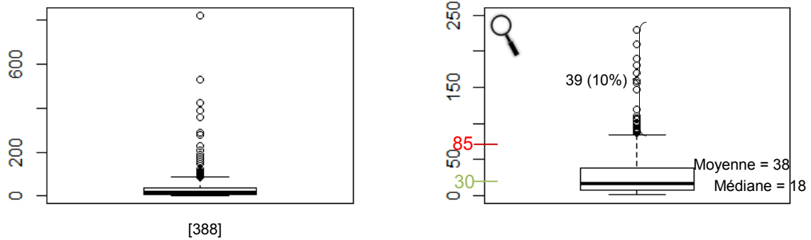
Figure 39 : Distribution des concentrations (en mg/L) du paramètre MES pour la famille CFI (à gauche) et zoom de 0 à 250 mg/L (à droite)
