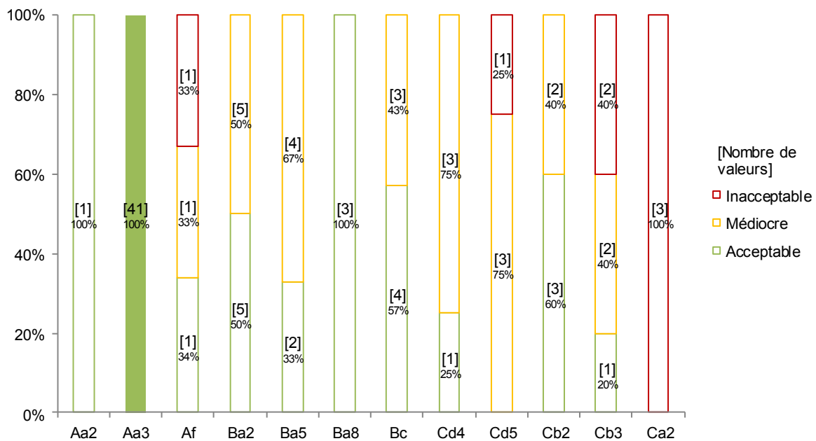
Figure 54 : Répartition dans chaque classe de qualité, selon les dispositifs, des paramètres azotés
