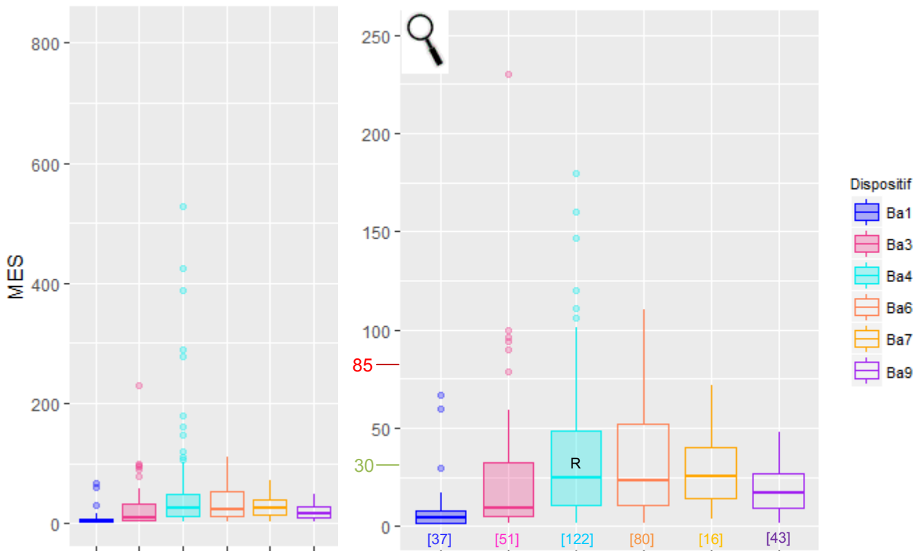
Figure 42 : Distribution des concentrations (en mg/L) du paramètre MES selon les dispositifs de la famille CFI (à gauche) et zoom de 0 à 250 mg/L (à droite)
