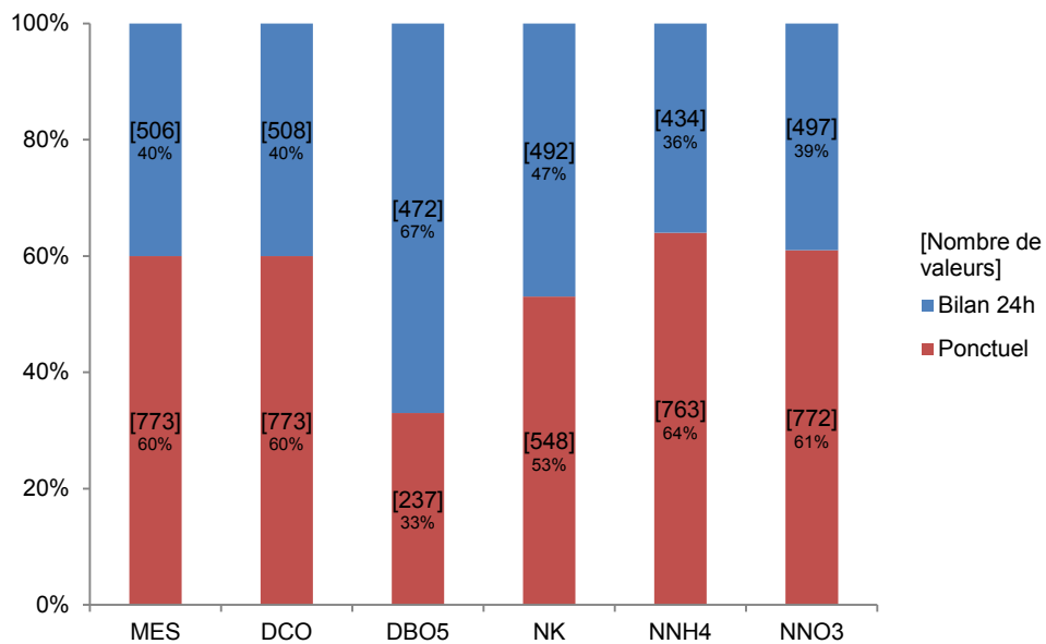
Figure 1 : Proportion de chaque paramètre chimique par type de prélèvements
