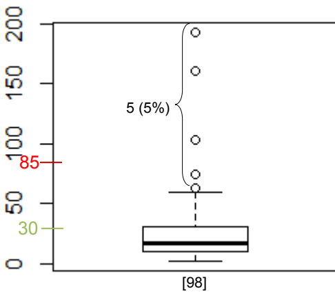
Figure 14: Distribution de toutes les concentrations (en mg/L) du paramètre MES pour la famille CFSF
