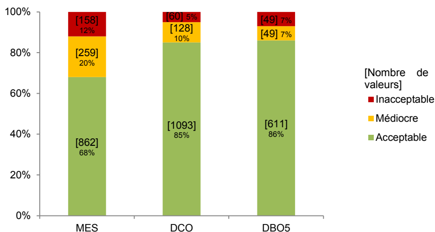
Figure 22 : Répartition, dans chaque classe de qualité, des trois paramètres MES, DCO et DBO 5 (ensemble des données)
