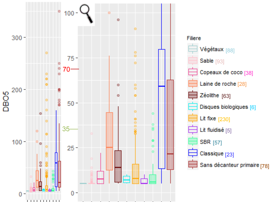
Figure 104: Distribution des concentrations (en mg/L) du paramètre DBO 5 selon les filières (à gauche) et zoom de 0 à 100 mg/L (à droite)
