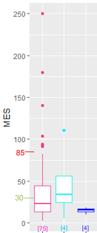
Figure 26 : Distribution des concentrations (en mg/L) du paramètre MES selon les filières de la famille CFI
