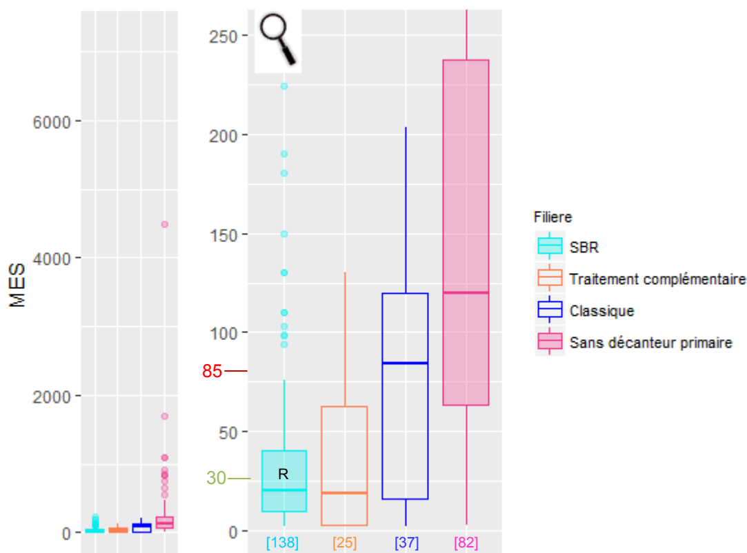
Figure 51 : Distribution des concentrations (mg/L) du paramètre MES selon les filières de la famille CL (à gauche) et zoom de 0 à 250 mg/L (à droite)
