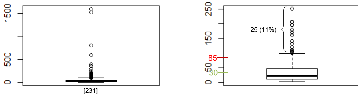
Figure 5 : Distribution de toutes les concentrations (en mg/L) du paramètre MES (à gauche) et zoom de 0 à 250 mg/L (à droite)
