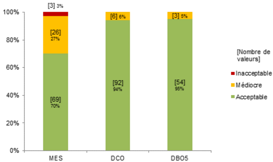
Figure 16 : Répartition, dans chaque classe de qualité, des trois paramètres MES, DCO et DBO 5 (famille CFSF)
