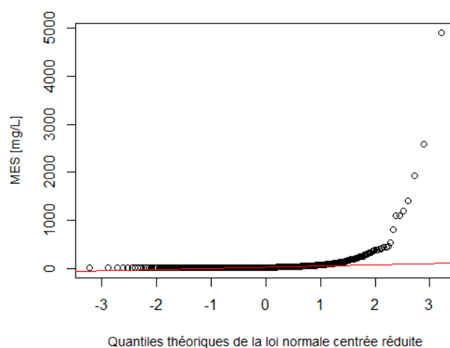
Figure 17 : Comparaison de la distribution empirique des MES à une loi normale centrée réduite
