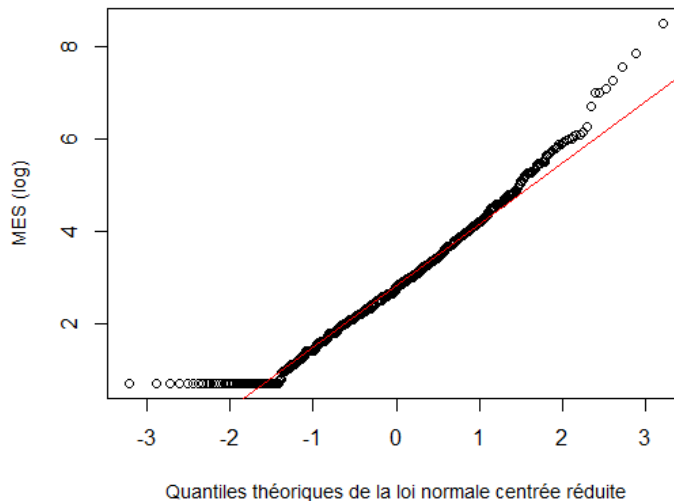
Figure 18 : Comparaison de la distribution empirique des MES (en ln) à une loi normale
