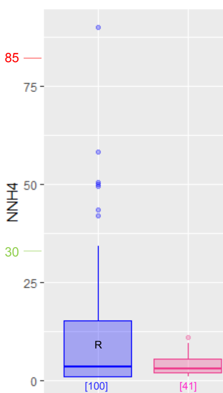
Figure 67 : Distribution des concentrations (en mg/L) du paramètre N-NH 4 + selon les dispositifs de la filière « sable »
