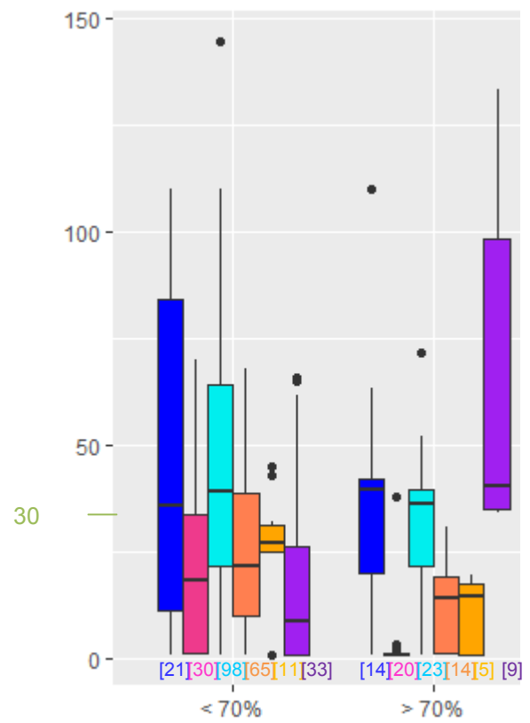
Figure 88 : Distribution des concentrations (en mg/L) du paramètre N-NO_3^- selon les dispositifs de la filière « lit fixe » et le taux de charge
