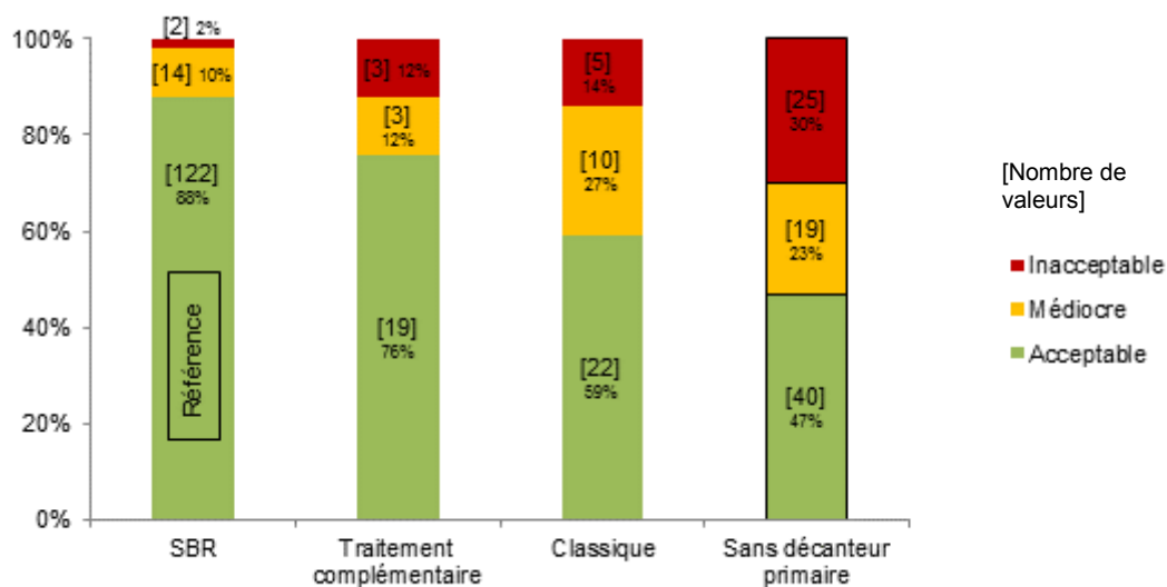
Figure 54 : Répartition dans chaque classe de qualité, selon les filières de la famille CL, du paramètre DCO
