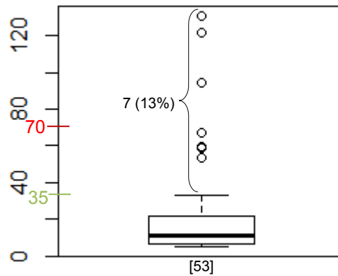
Figure 24 : Distribution de toutes les concentrations (en mg/L) du paramètre DBO 5 pour la famille CFI
