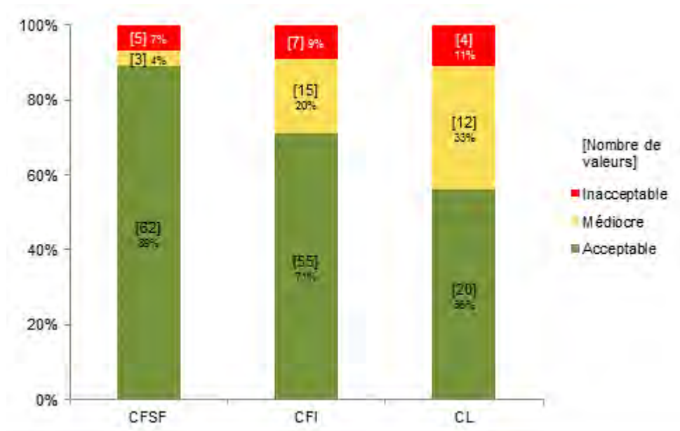
Figure 121: Répartition des installations par famille selon leurs fréquences « acceptable », « médiocre » ou « inacceptable » de l'entretien « curatif »
