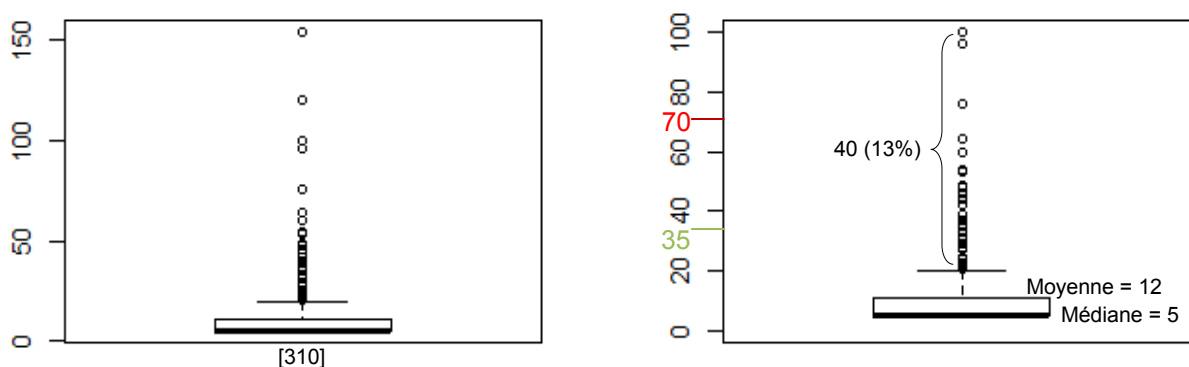
Figure 29 : Distribution des concentrations (en mg/L) du paramètre DBO 5 pour la famille CFSF (à gauche) et zoom de 0 à 100 mg/L (à droite)
