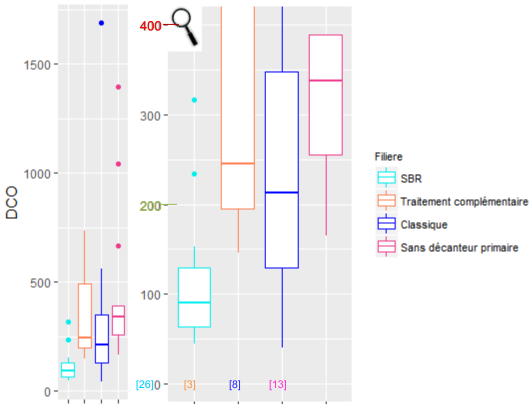
Figure 37: Distribution des concentrations (en mg/L) du paramètre DCO selon les filières de la famille CL (à gauche) et zoom de 0 à 400 mg/L (à droite)
