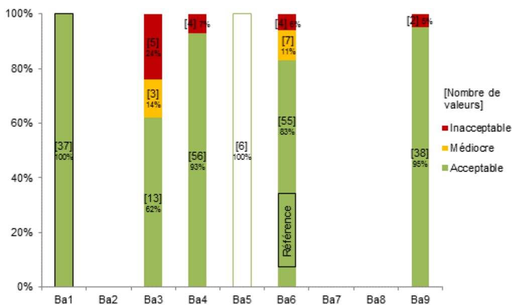
Figure 47 : Répartition dans chaque classe de qualité, selon les dispositifs de la filière « lit fixe », du paramètre DBO_5
