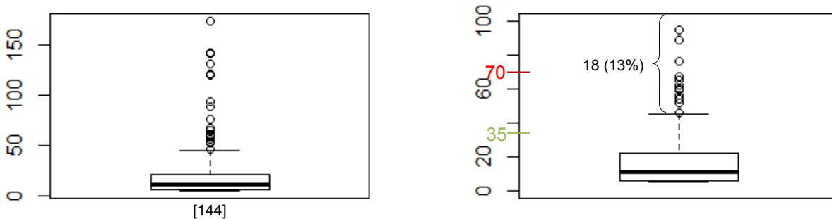
Figure 6 : Distribution de toutes les concentrations (en mg/L) du paramètre DBO 5 (à gauche) et zoom de 0 à 100 mg/L (à droite)
