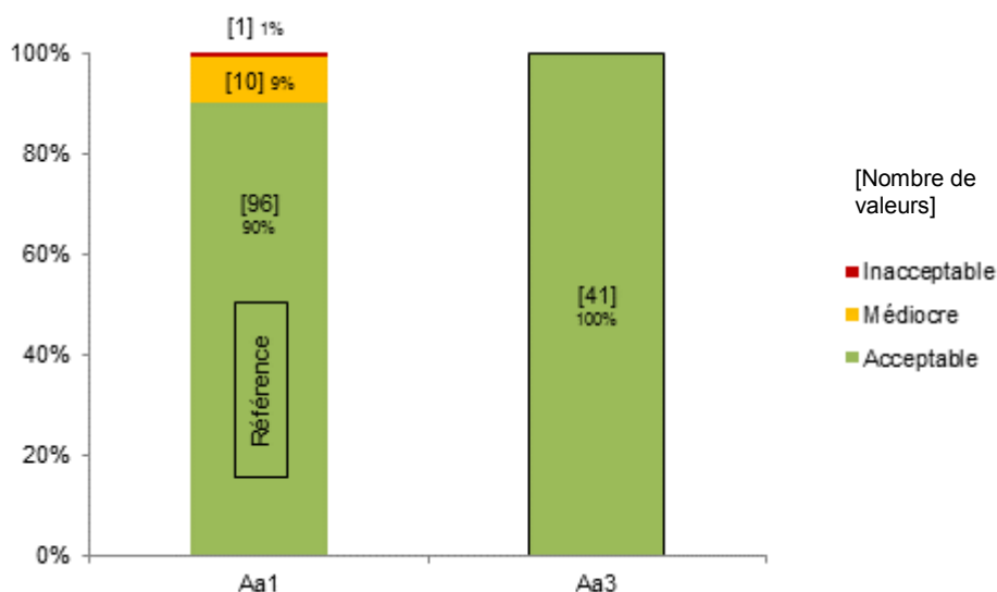
Figure 69 : Répartition dans chaque classe de qualité, selon les dispositifs de la filière « sable », des paramètres caractéristiques de l'azote
