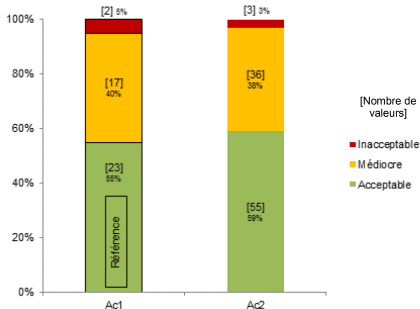
Figure 71 : Répartition dans chaque classe de qualité, selon les dispositifs de la filière « zéolithe », des paramètres caractéristiques de l'azote
