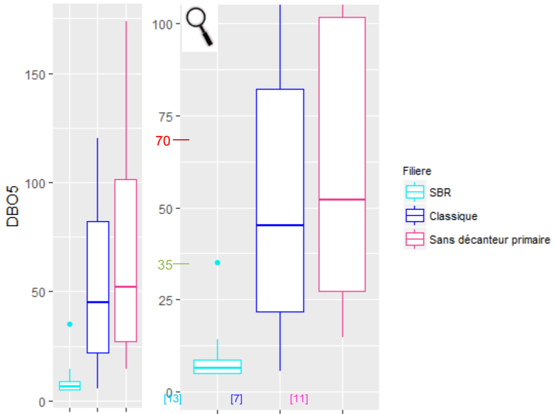
Figure 39 : Distribution des concentrations (en mg/L) du paramètre DBO 5 selon les filières de la famille CL (à gauche) et zoom de 0 à 100 mg/L (à droite)
