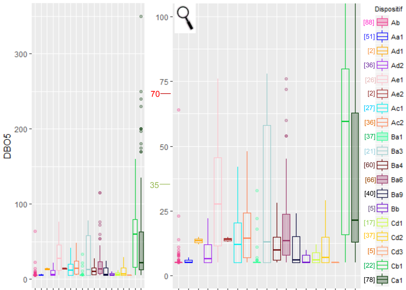
Figure 114 : Distribution des concentrations (en mg/L) du paramètre DBO 5 selon les dispositifs (à gauche) et zoom de 0 à 100 mg/L (à droite)
