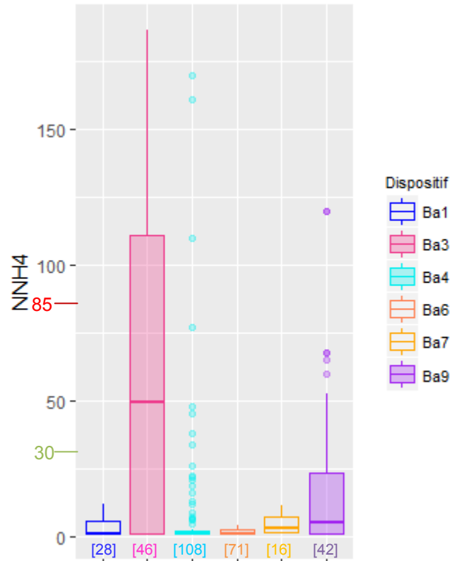
Figure 86 : Distribution des concentrations (en mg/L) du paramètre N-NH_4^+ selon les dispositifs de la filière « lit fixe »
