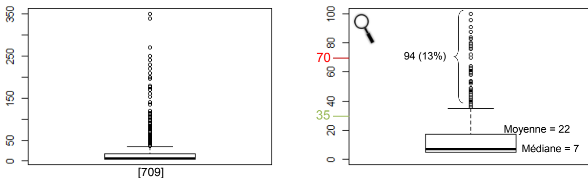
Figure 21 : Distribution de toutes les concentrations (en mg/L) du paramètre DBO 5 (à gauche) et zoom de 0 à 100 mg/L (à droite)
