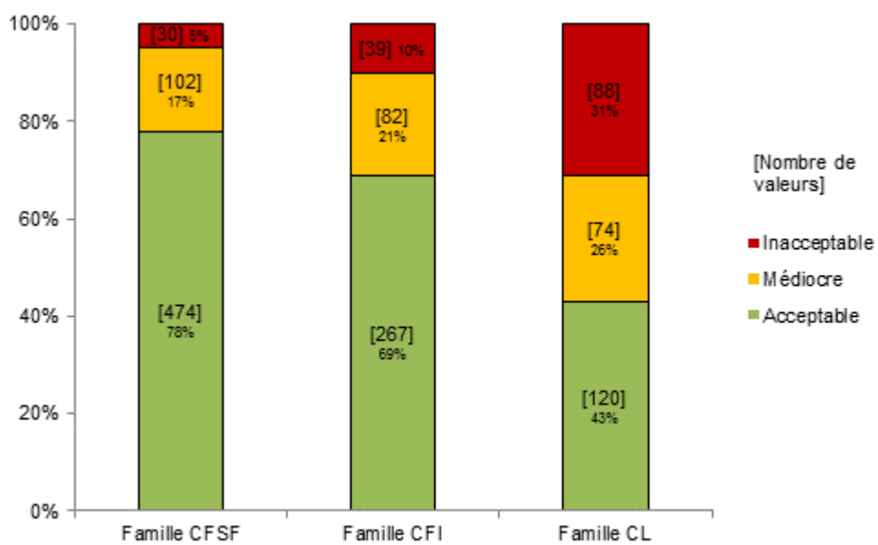
Figure 91 : Répartition dans chaque classe de qualité, selon les familles, du paramètre chimique MES
