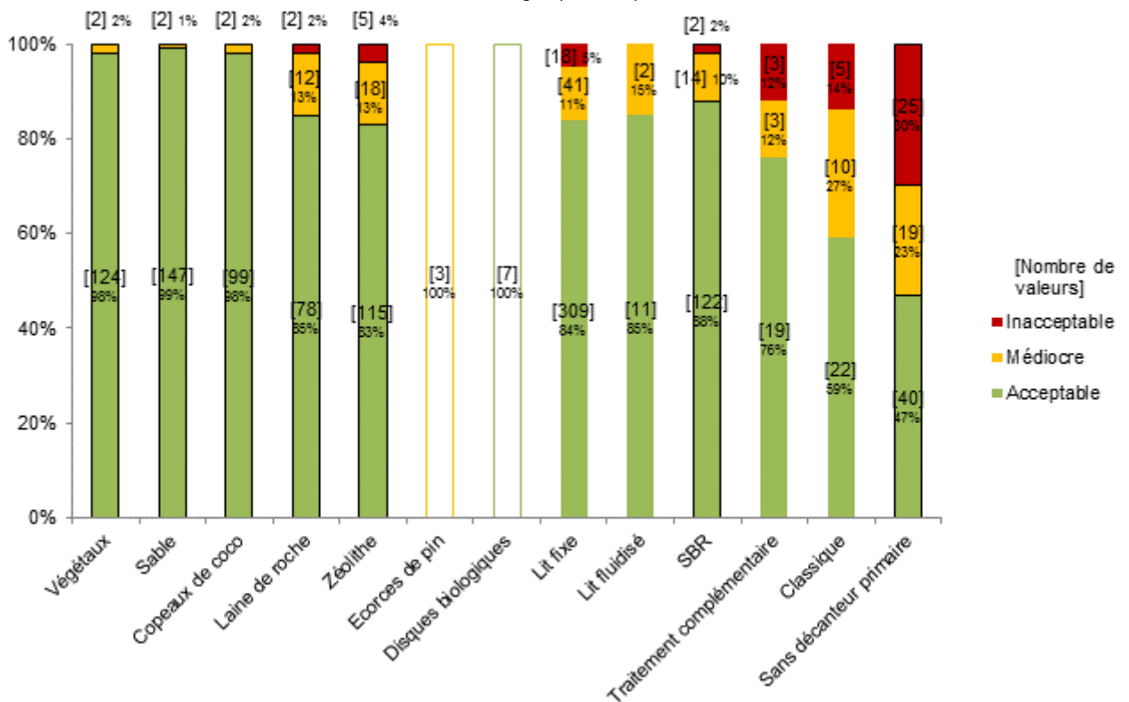
Figure 103 41 : Répartition dans chaque classe de qualité, selon les filières, du paramètre DCO
