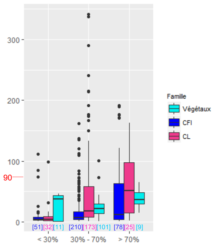
Figure 78 : Distribution des concentrations (en mg/L) du paramètre chimique NK selon les familles et le taux de charge
