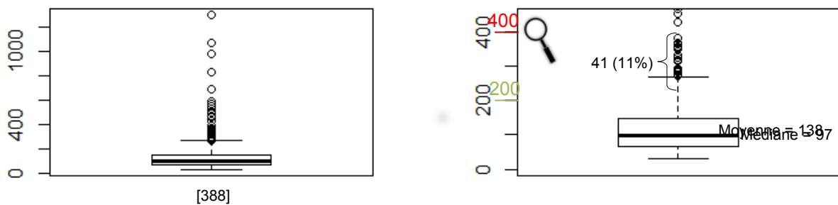
Figure 40 : Distribution des concentrations (en mg/L) du paramètre DCO pour la famille CFI (à gauche) et zoom de 0 à 400 mg/L (à droite)
