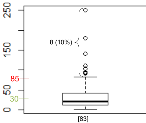
Figure 23 : Distribution de toutes les concentrations (en mg/L) du paramètre MES pour la famille CFI
