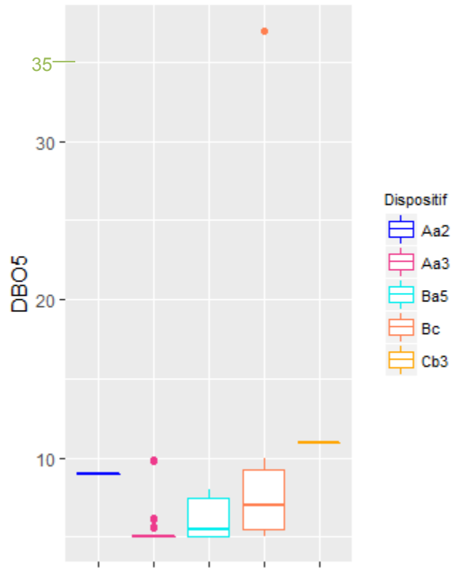
Figure 49 : Distribution des concentrations (en mg/L) du paramètre DBO 5 selon les dispositifs
