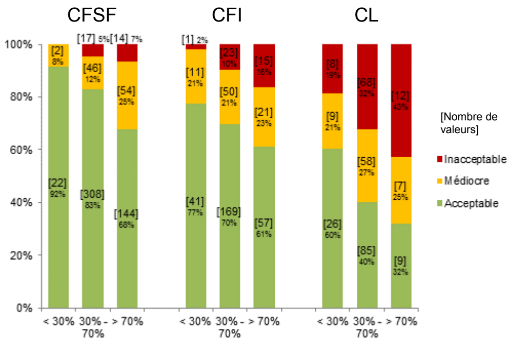
Figure 1 : Répartition dans chaque classe de qualité, selon taux de charge et familles, du paramètre MES
