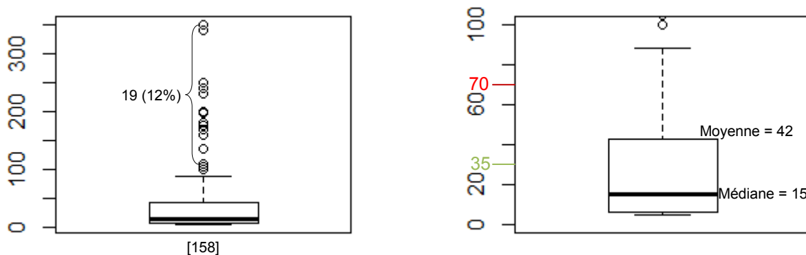
Figure 49 : Distribution des concentrations (en mg/L) du paramètre DBO 5 de la famille CL (à gauche) et zoom de 0 à 100 mg/L (à droite)
