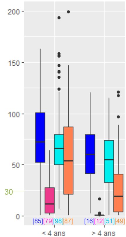
Figure 64 : Distribution des concentrations (en mg/L) du paramètre N-NO_3^- pour les dispositifs nitrifiants et selon l'âge
