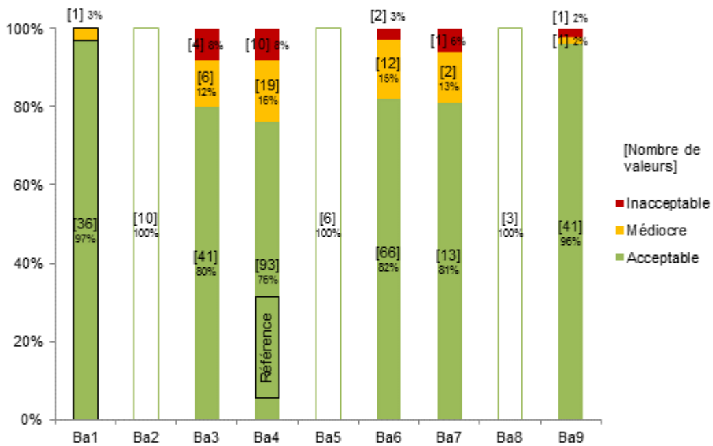
Figure 45 : Répartition dans chaque classe de qualité, selon les dispositifs de la filière « lit fixe », du paramètre DCO
