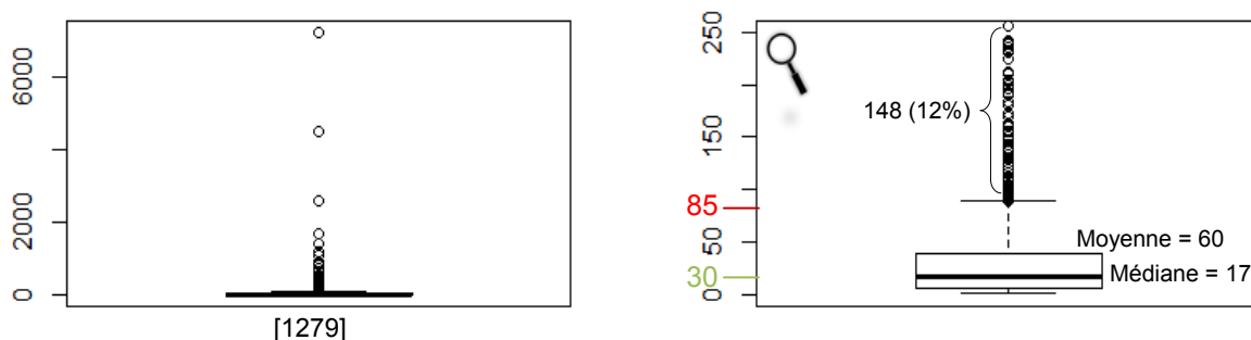
Figure 20 : Distribution de toutes les concentrations (en mg/L) du paramètre MES (à gauche) et zoom de 0 à 250 mg/L (à droite)
