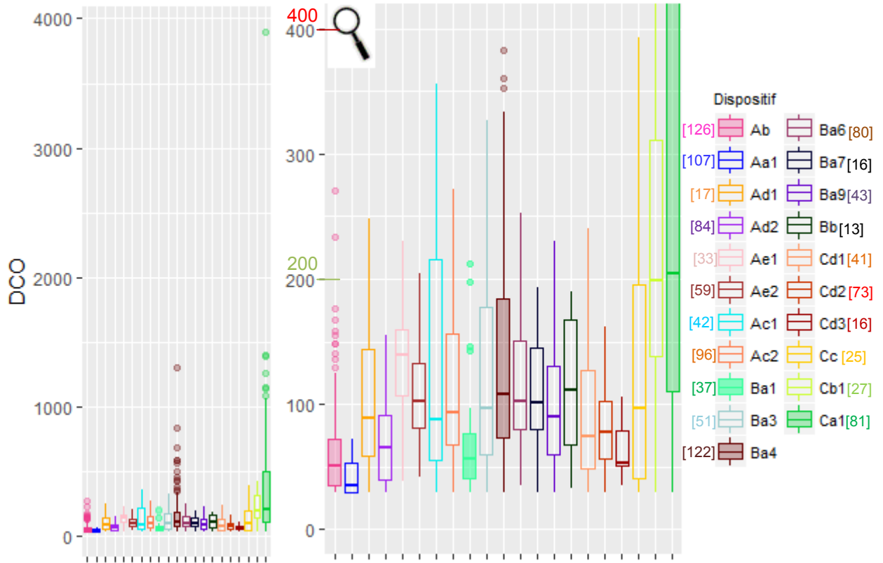
Figure 112 : Distribution des concentrations (en mg/L) du paramètre DCO selon les dispositifs (à gauche) et zoom de 0 à 400 mg/L (à droite)
