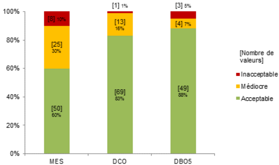
Figure 25 : Répartition, dans chaque classe de qualité, des trois paramètres MES, DCO et DBO 5 (famille CFI)
