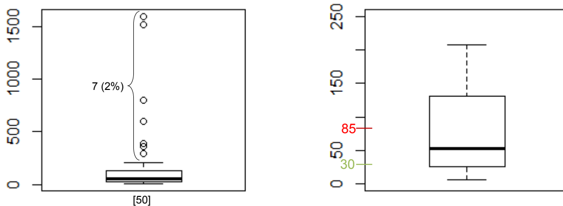
Figure 32 : Distribution de toutes les concentrations (en mg/L) du paramètre MES de la famille CL (à gauche) et zoom de 0 à 250 mg/L (à droite)
