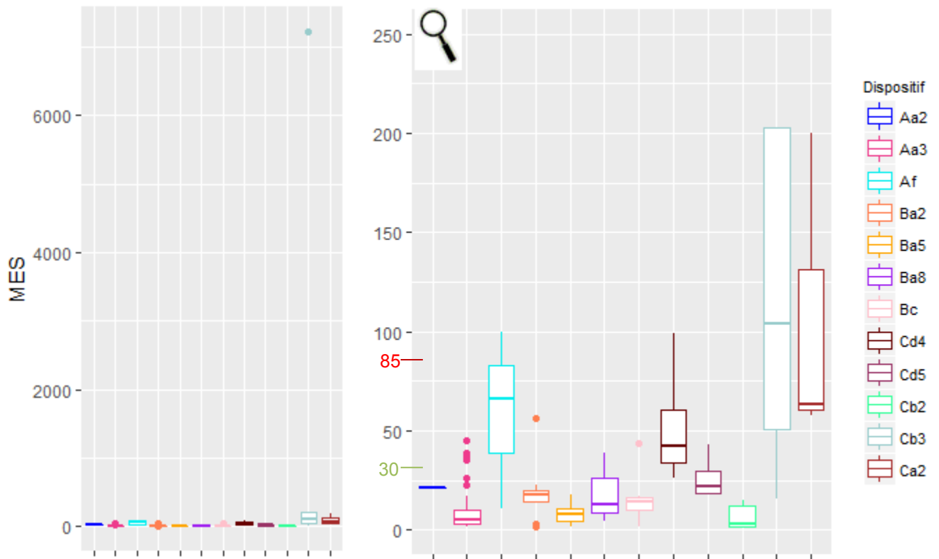
Figure 45 : Distribution des concentrations (en mg/L) du paramètre MES selon les dispositifs (à gauche) et zoom de 0 à 250 mg/L (à droite)
