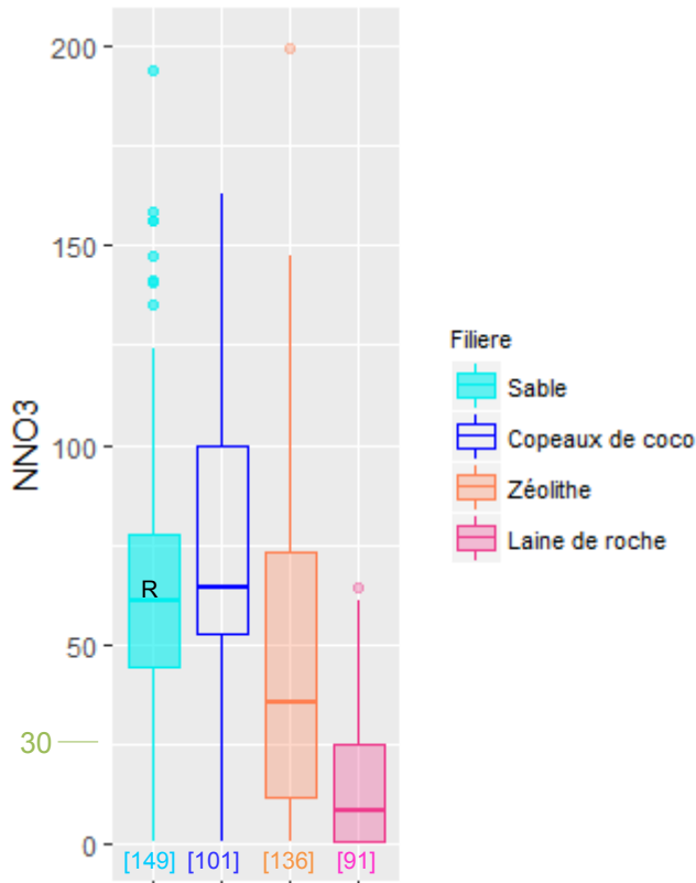
Figure 63 : Distribution des concentrations (en mg/L) du paramètre N-NO_3^- pour les dispositifs nitrifiants
