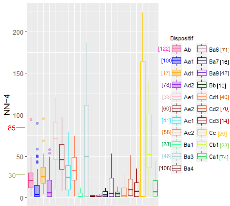
Figure 117 : Distribution des concentrations (en mg/L) du paramètre N-NH_4^+ selon les dispositifs
