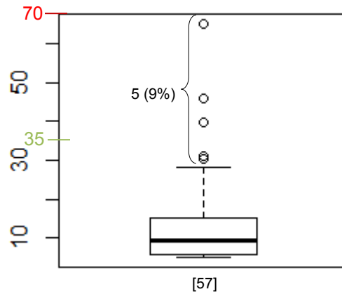
Figure 15: Distribution de toutes les concentrations (en mg/L) du paramètre DBO 5 pour la famille CFSF
