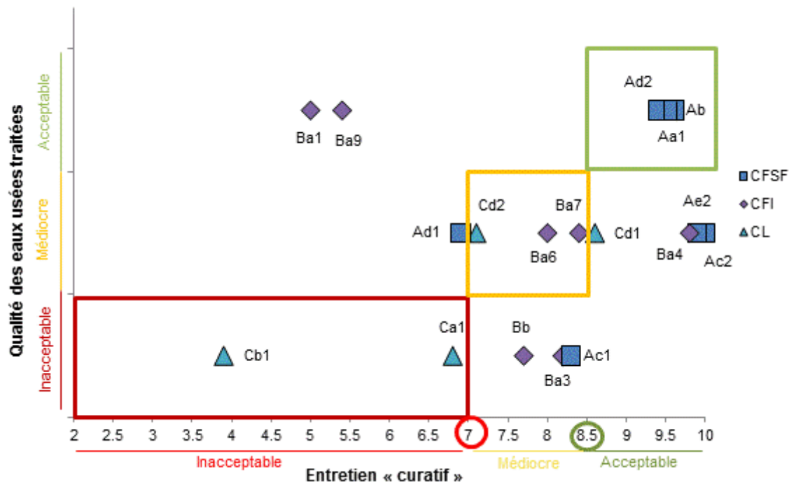
Figure 133 : Analyse conjointe de la qualité des eaux usées traitées et de l'entretien « curatif » de 18 dispositifs
