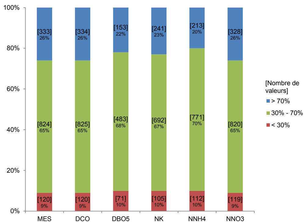
Figure 3 : Proportion de chaque paramètre chimique par taux de charge
