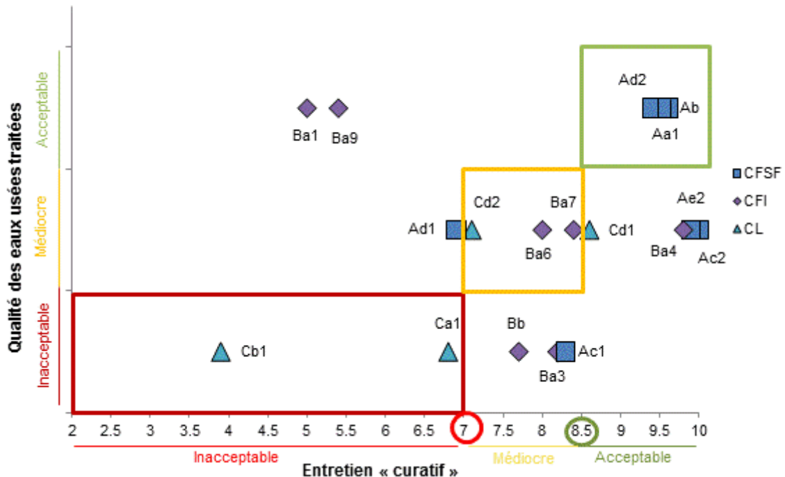
Figure 136 : Analyse conjointe de la qualité des eaux usées traitées et de l'entretien « curatif » des 18 dispositifs
