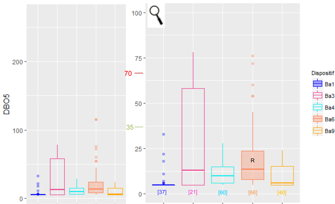
Figure 46 : Distribution des concentrations (en mg/L) du paramètre DBO_5 selon les dispositifs de la famille CFI (à gauche) et zoom de 0 à 100 mg/L (à droite)
