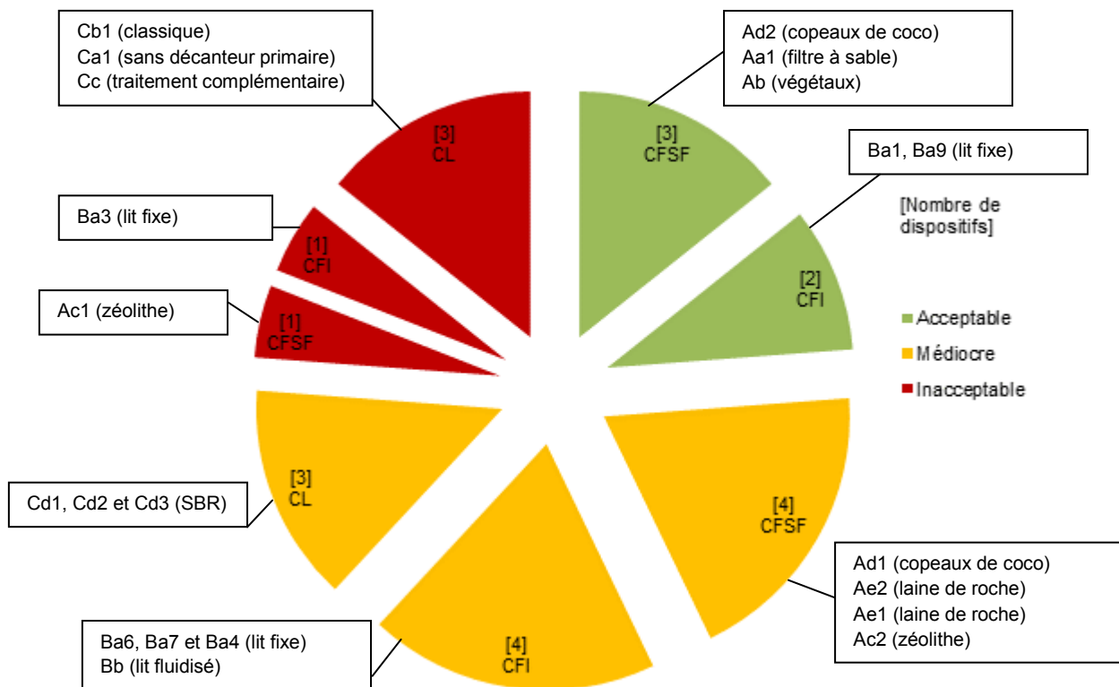
Figure 130 : Nombre de dispositifs par famille et par classe de qualité globale
