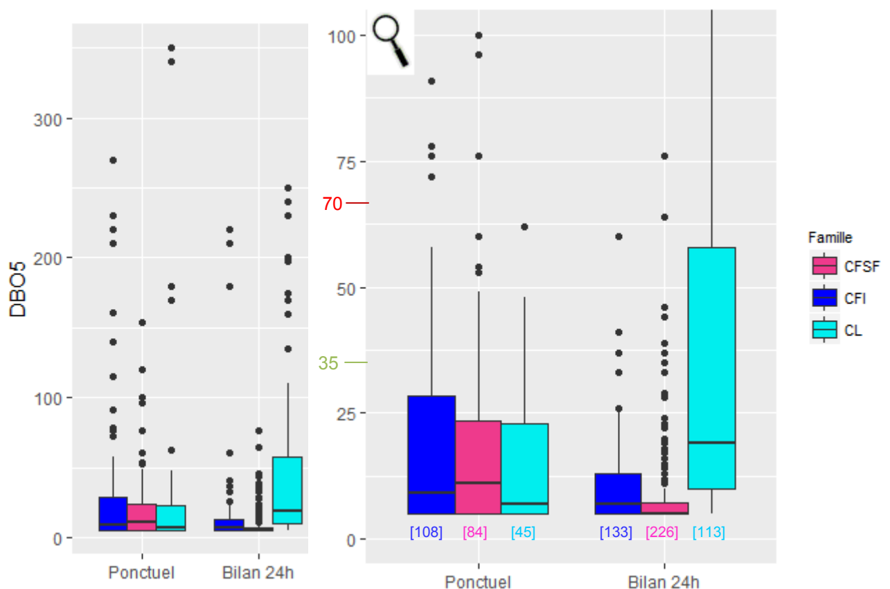
Figure 27 : Distribution des concentrations (en mg/L) du paramètre DBO 5 selon le type de prélèvement et par famille (à gauche) et zoom de 0 à 100 mg/L (à droite)
