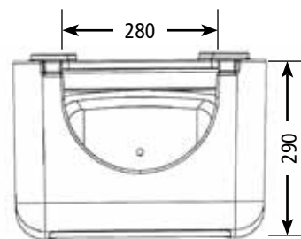
Armoire intérieure PPE vue du haut (Art. 35248).
