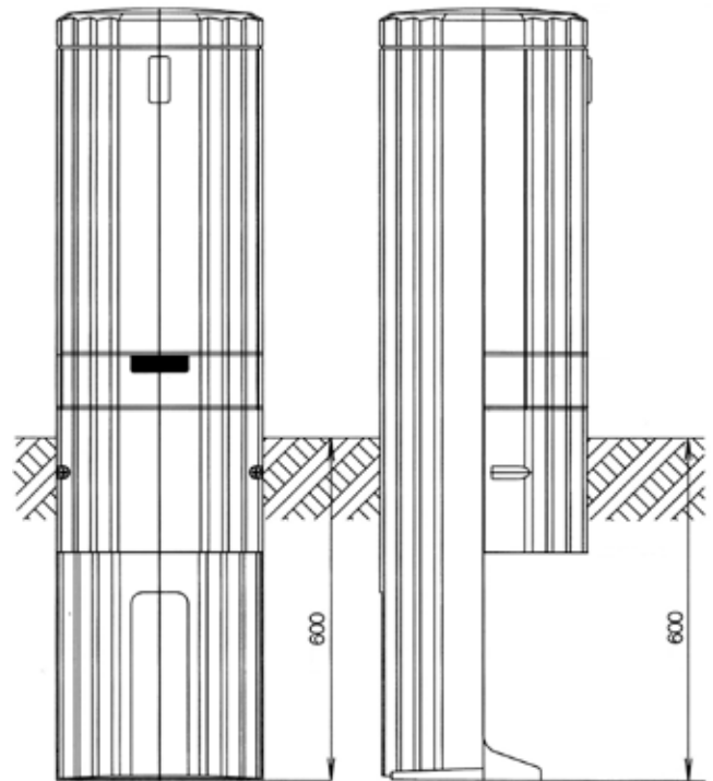
Dimensions de la colonne extérieure de l'armoire de commande extérieure plastique (Art. : 32733 - vendue séparément).
