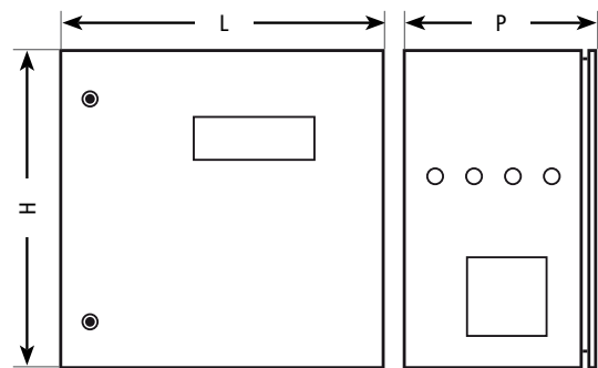
Dimensions de l'armoire intérieure métallique (Art. : 32470).
