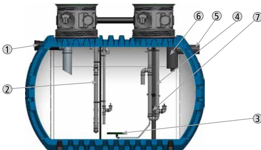
Vue de coupe d'une micro-station ACTIBLOC® 8EH (7000 DP).
