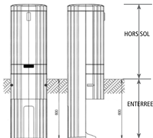
Dimensions de la colonne extérieure de l'armoire de commande extérieure plastique (Art. : 32733 - vendue séparément).
