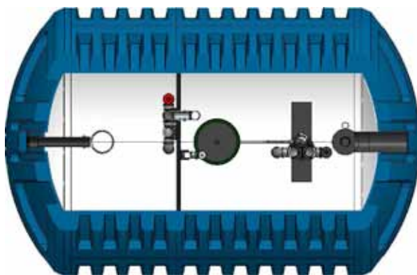
Vue de coupe d'une micro-station ACTIBLOC® 8EH (7000 DP).
