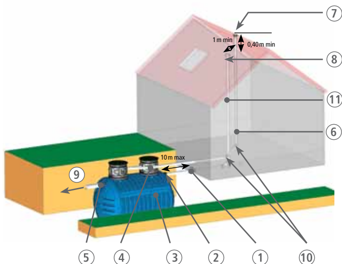
Schéma de raccordement de la ventilation haute pour une micro-station ACTIBLOC® 8EH (7000 DP).
